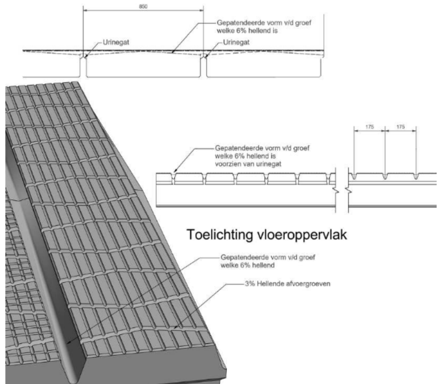
Abbeeldingen vloerelementen en de gieraafvoer
