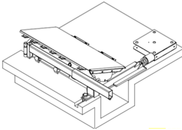
Detail mestafstort BWL 2013.04.V5
