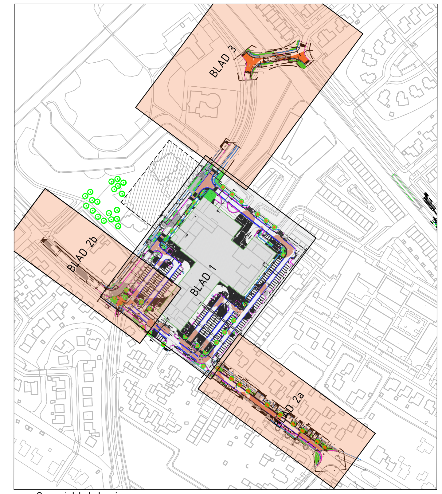
Overzicht tekening Schaal 1:2500
