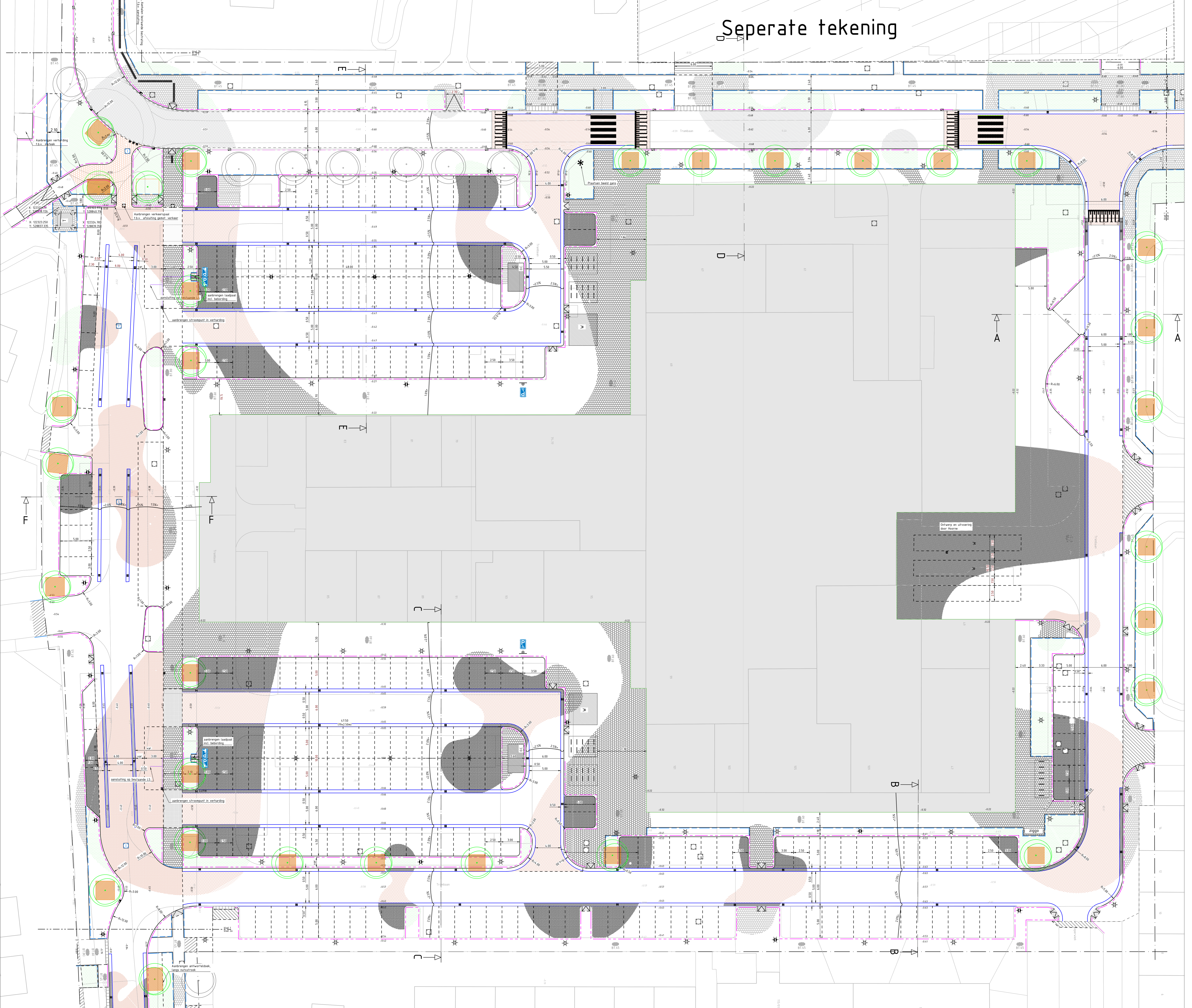
Situatie tekening, blad 1 Schaal 1:200
