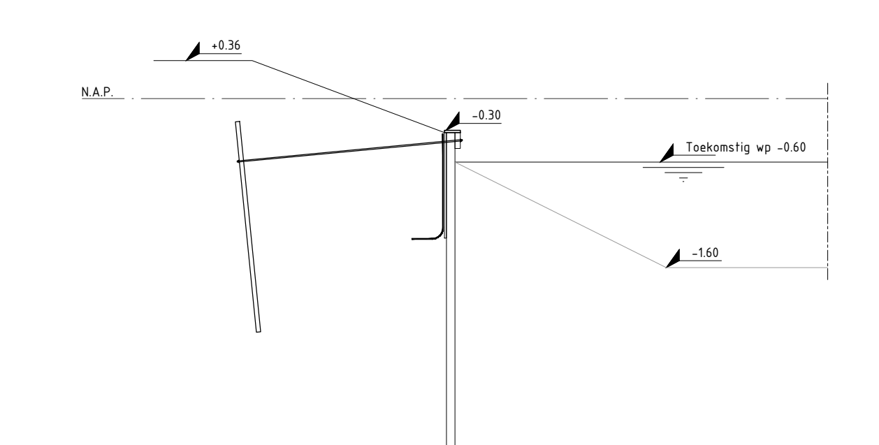
Principedetail 3, definitieve situatie met waterpeil 0.60-NAP Schaal 1:50
