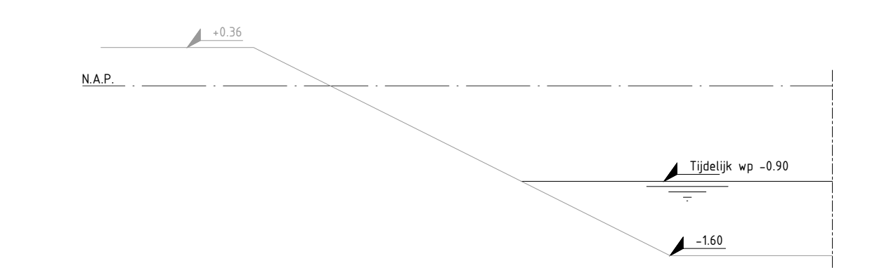
Principedetail 1, bestaande situatie met tijdelijk waterpeil 0.90-NAP Schaal 1:50
