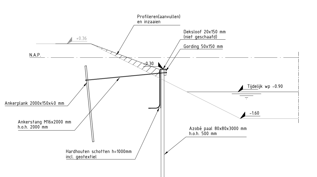
Principedetail 2, tijdelijke situatie met beschoeiing, waterpeil 0.90-NAP Schaal 1:50
