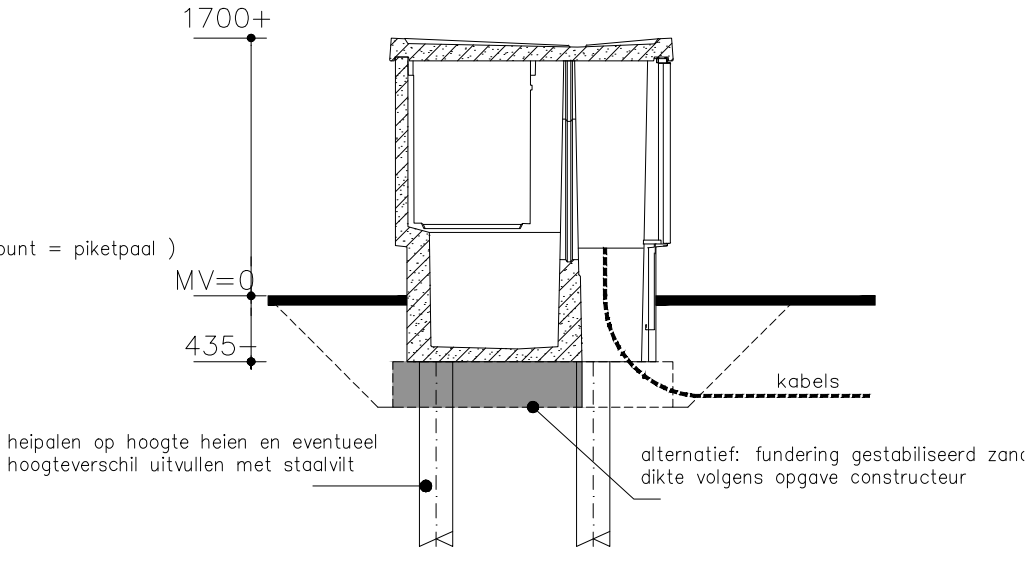
DOORSNEDE A-A
