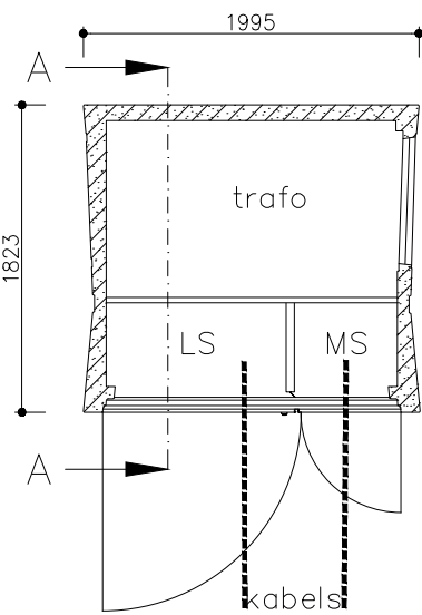
PLATTEGROND
