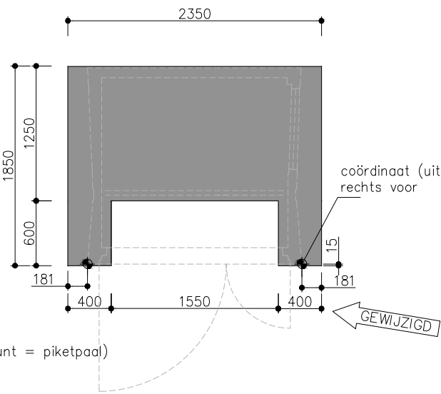
FUNDERING GESTABILISEERD ZAND dikte volgens opgave constructeur
