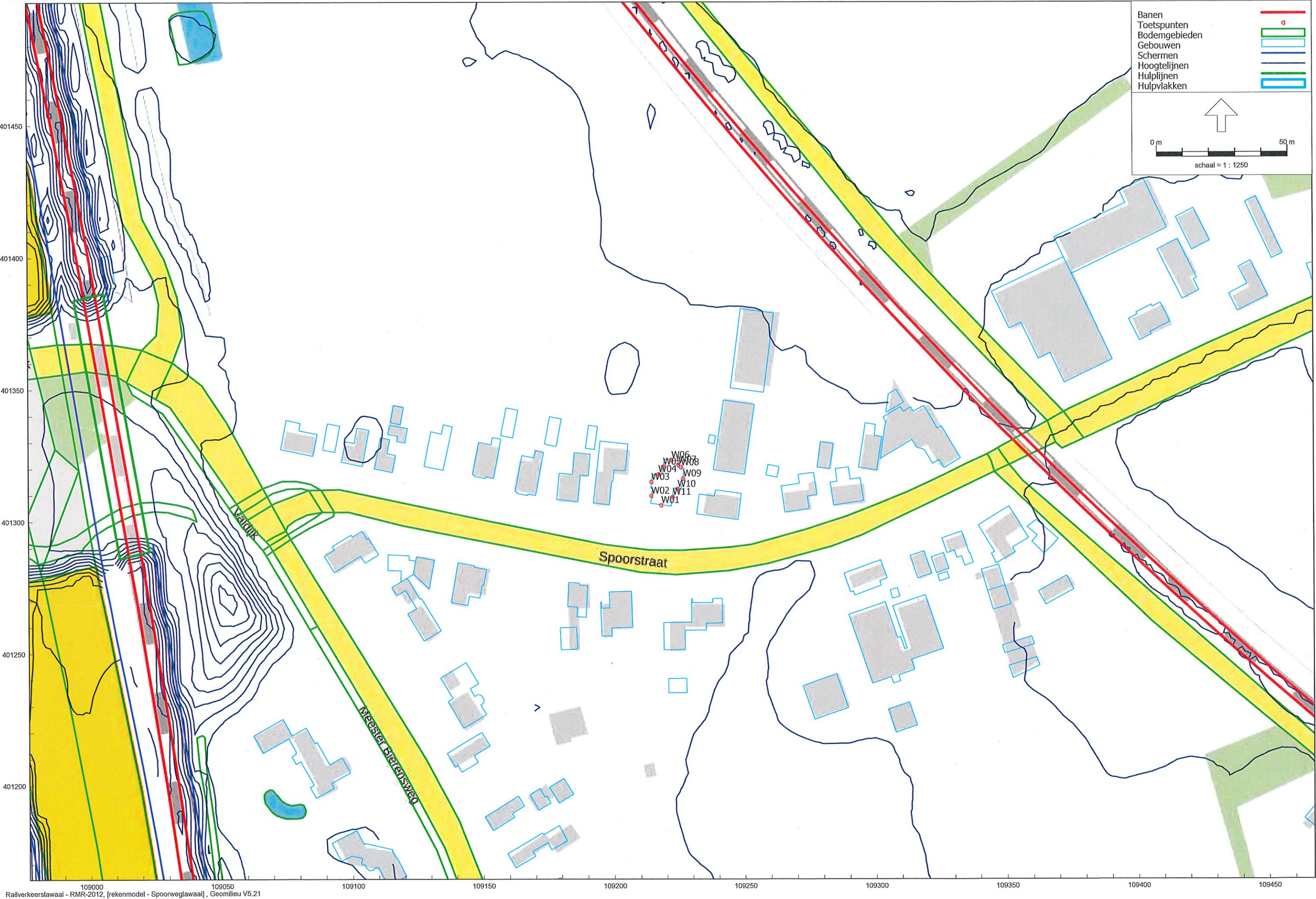
Figuur 3C: overzicht modellering railverkeerslawaaï
