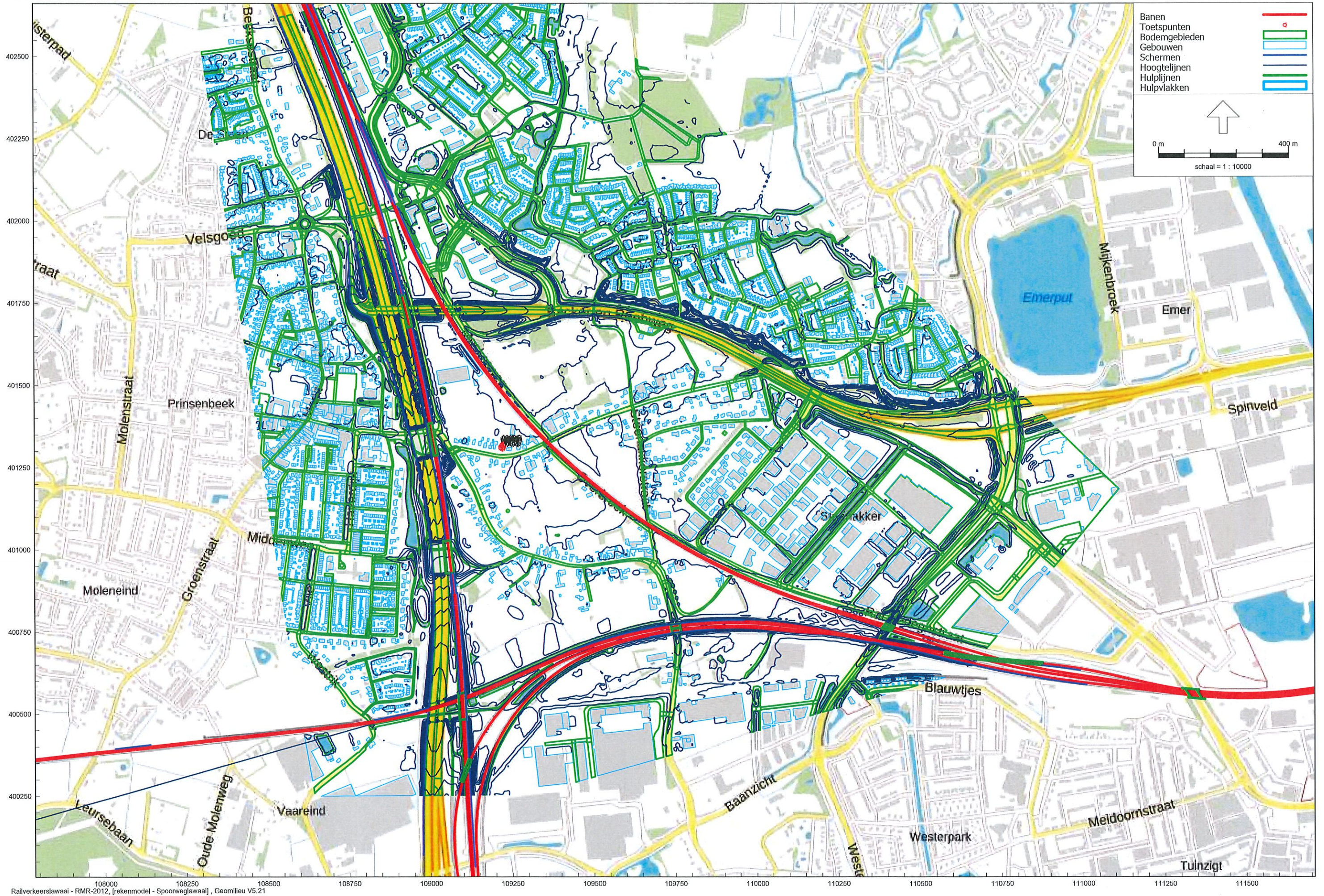
Figuur 3B: overzicht modellering railverkeerslawaaai
