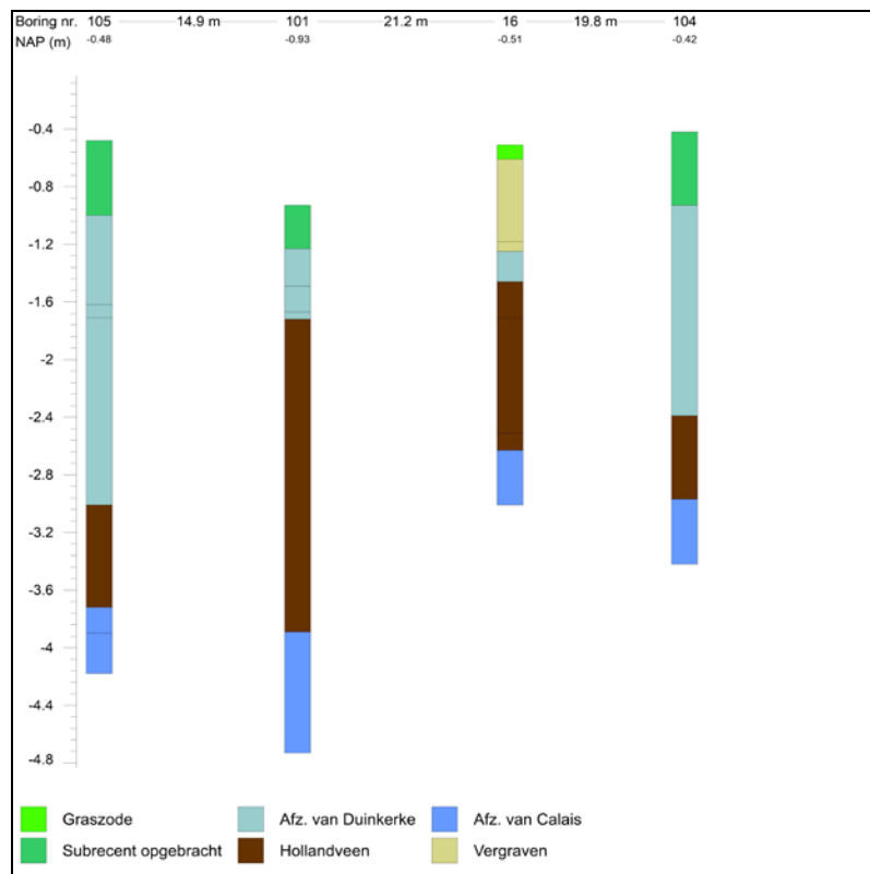
Afbeelding 33. Grafische weergave van Boring nr. 105, 101, 16 en 104.
