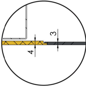
Section „B-B“ Detail
