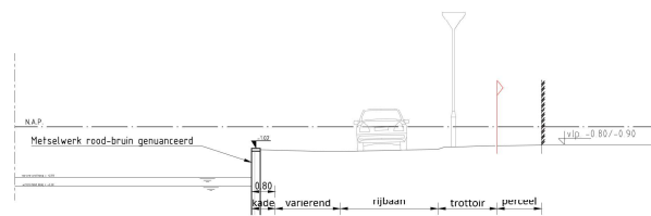
■ Principeprofiel 9: Kademuur
