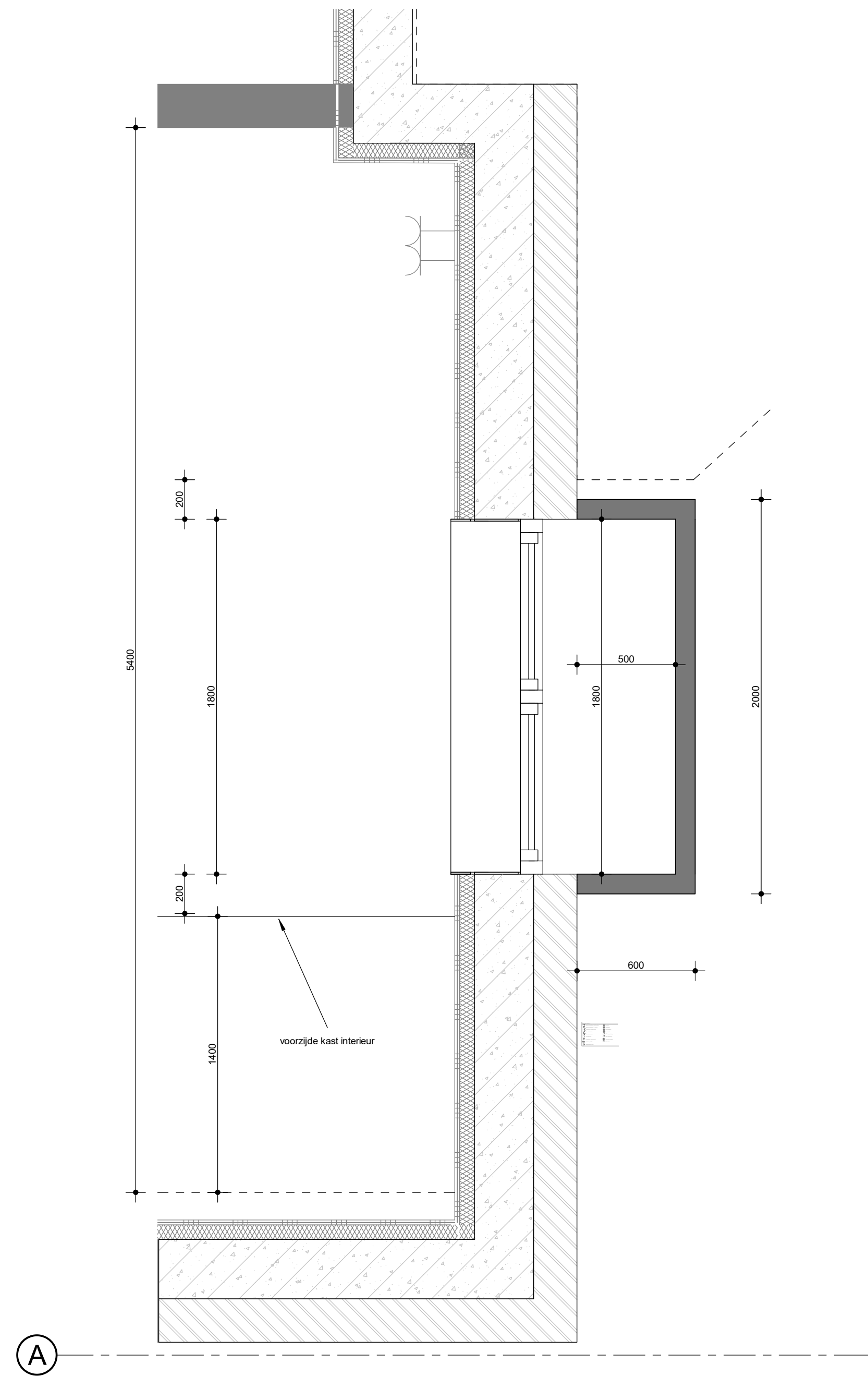
-1 kelder nieuw - Callout 1 doorsnede schaal 1 : 20
