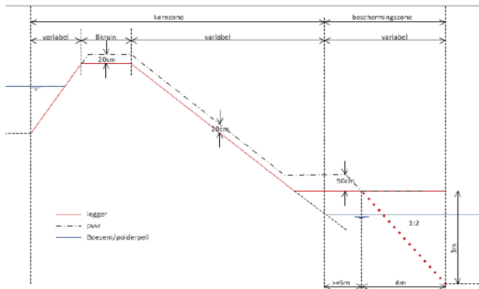
figuur: Zonering van de waterkering
