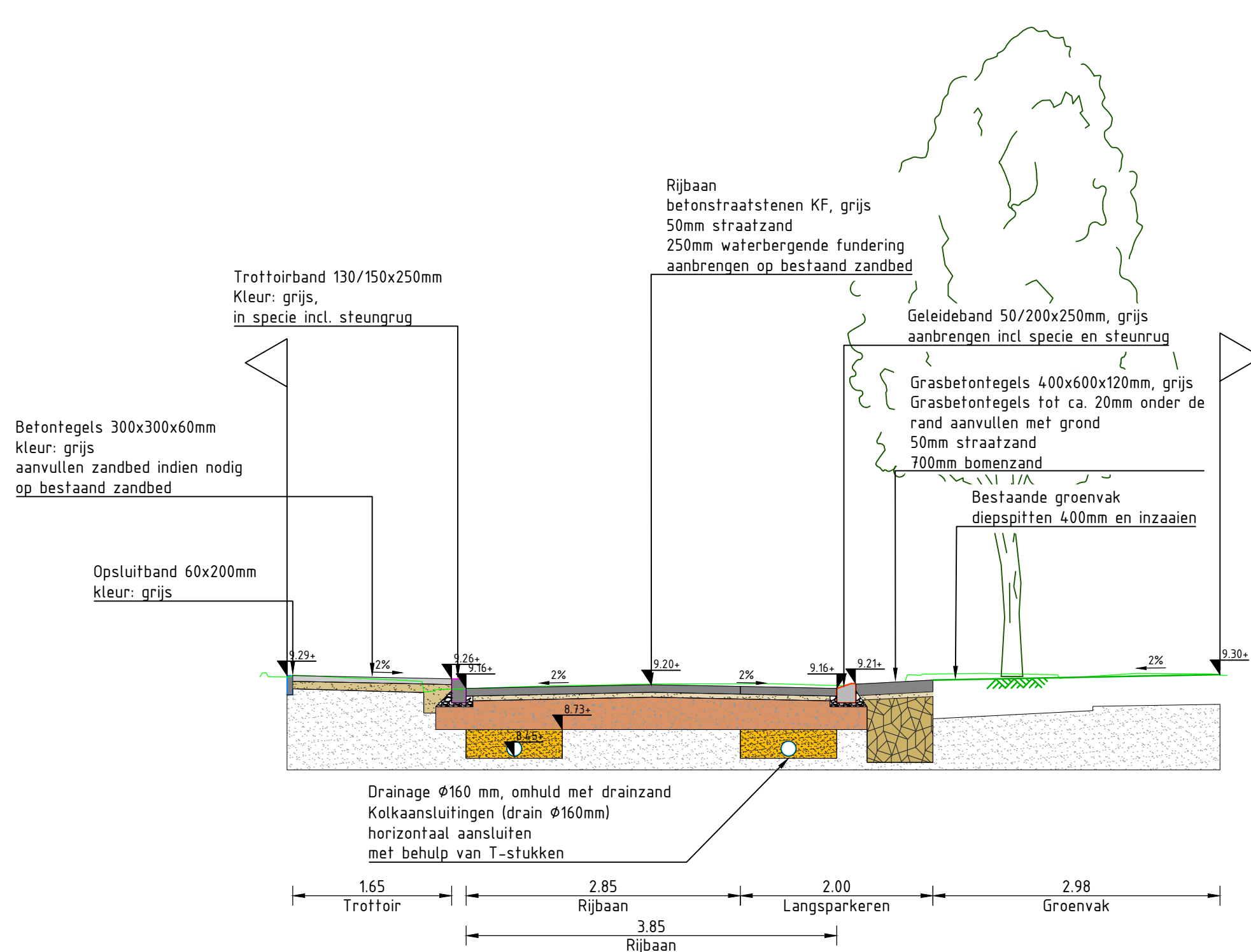
Dwarsprofiel B-B
