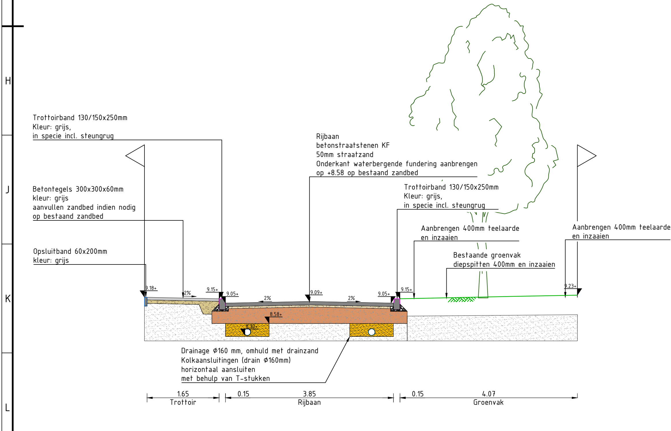
Dwarsprofiel A-A
