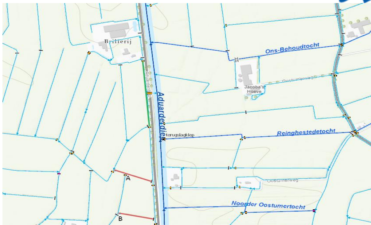
Figuur 1: Locatie van werkzaamheden. Rode lijnen geven de te dempen watergangen weer. De groen lijn geeft de te verbreden watergang weer.
