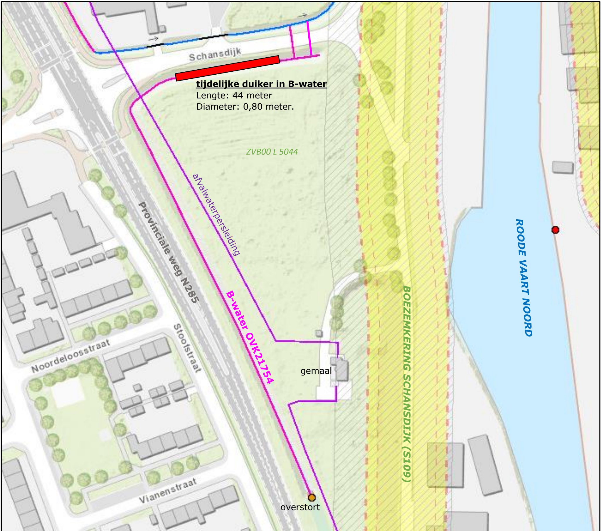
317983-A Topografische situatie
