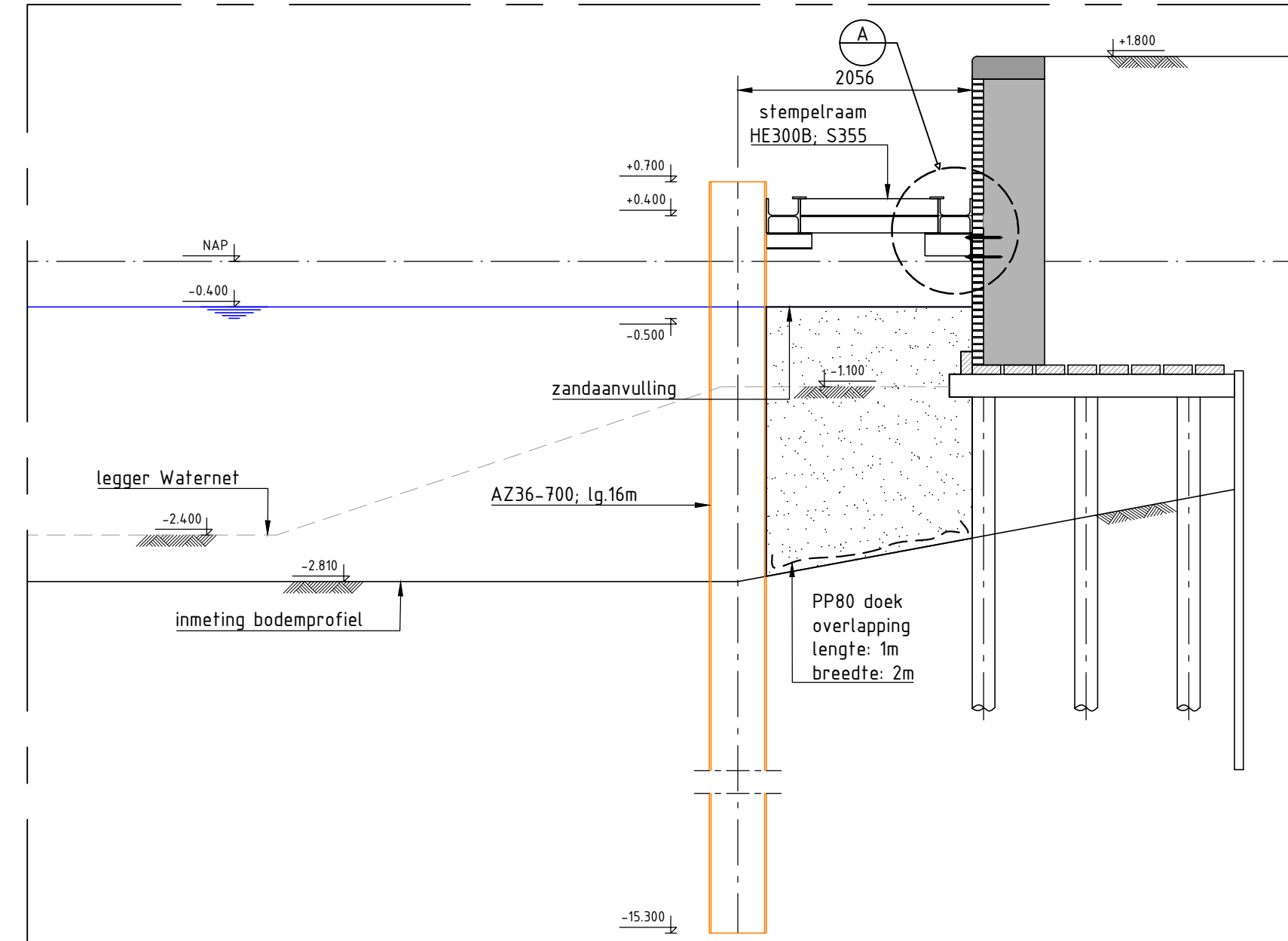
DOORSNEDE A-A
