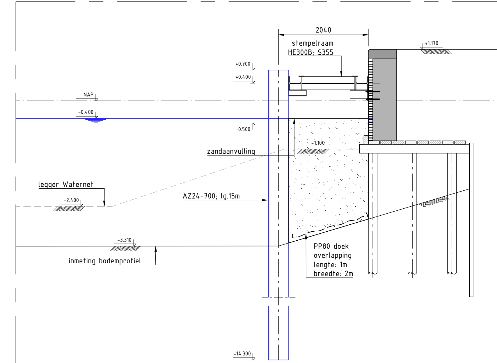
DOORSNEDE B-B
