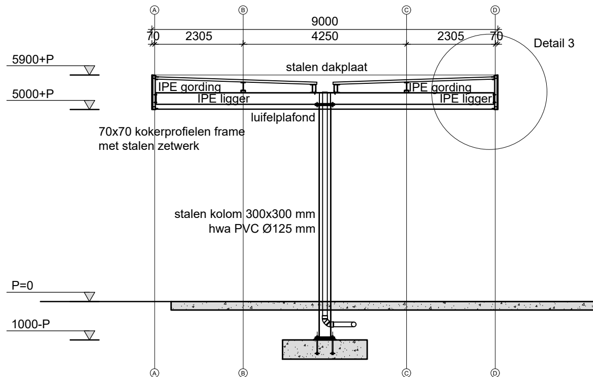
Principe dwarsdoorsnede: Luifel en fundering Schaal 1:100
