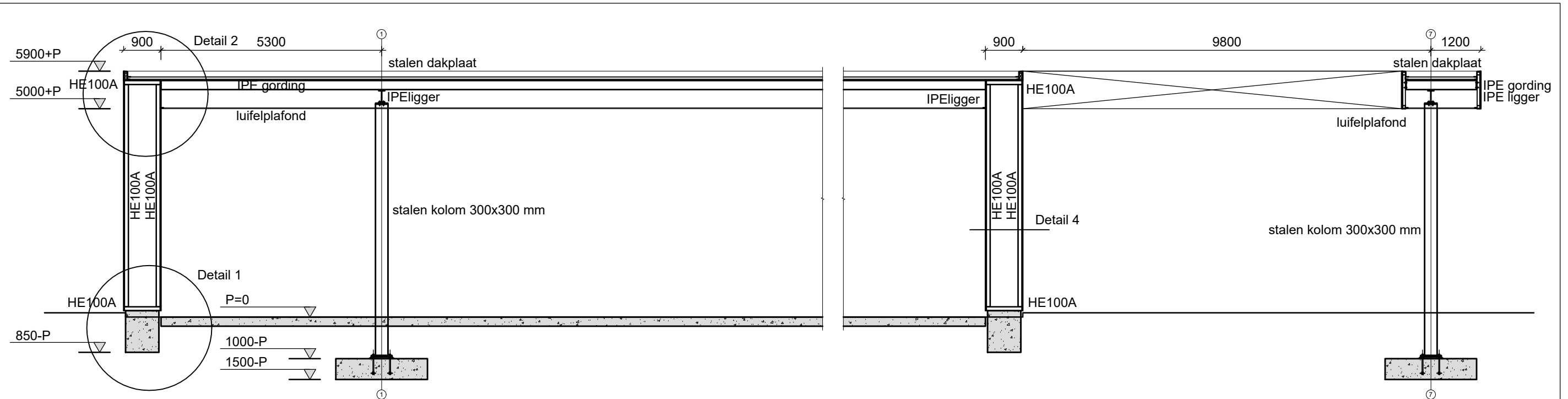
Principe langsdoorsnede: Luifel en fundering Schaal 1:100
