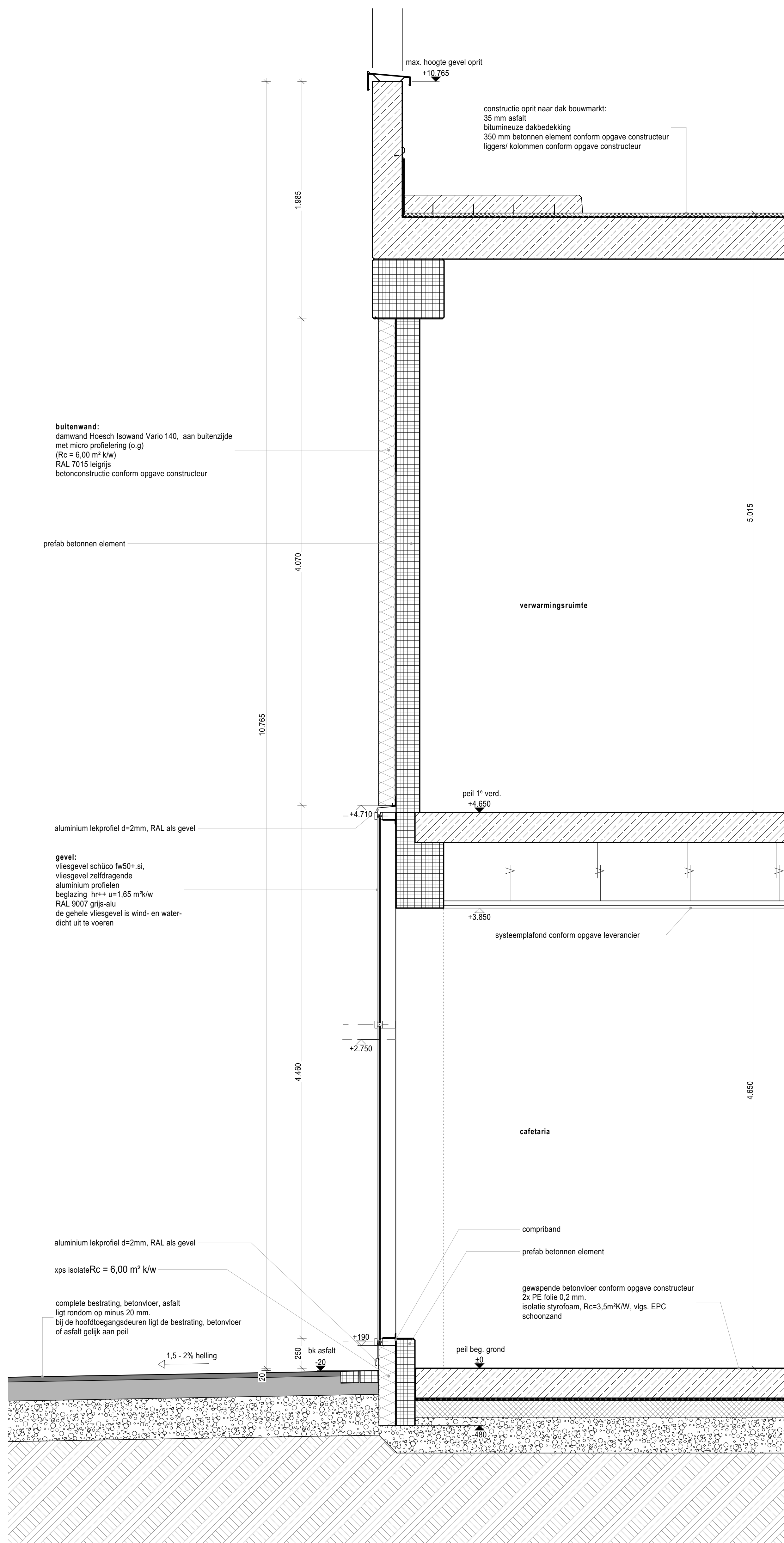
VERTICALE DOORSNEDE (s. 1:20)
