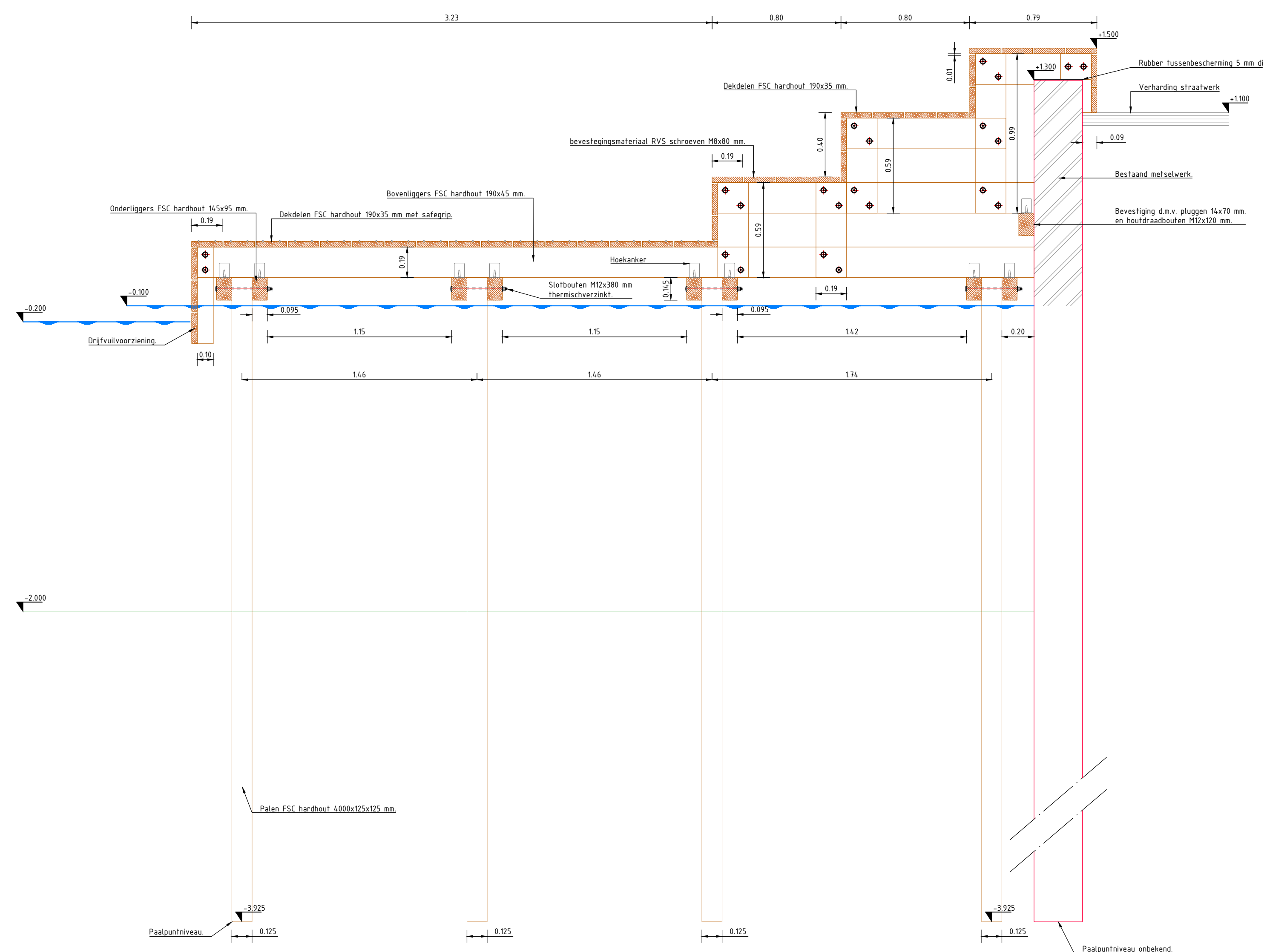
Doorsnede 2. 1:20
