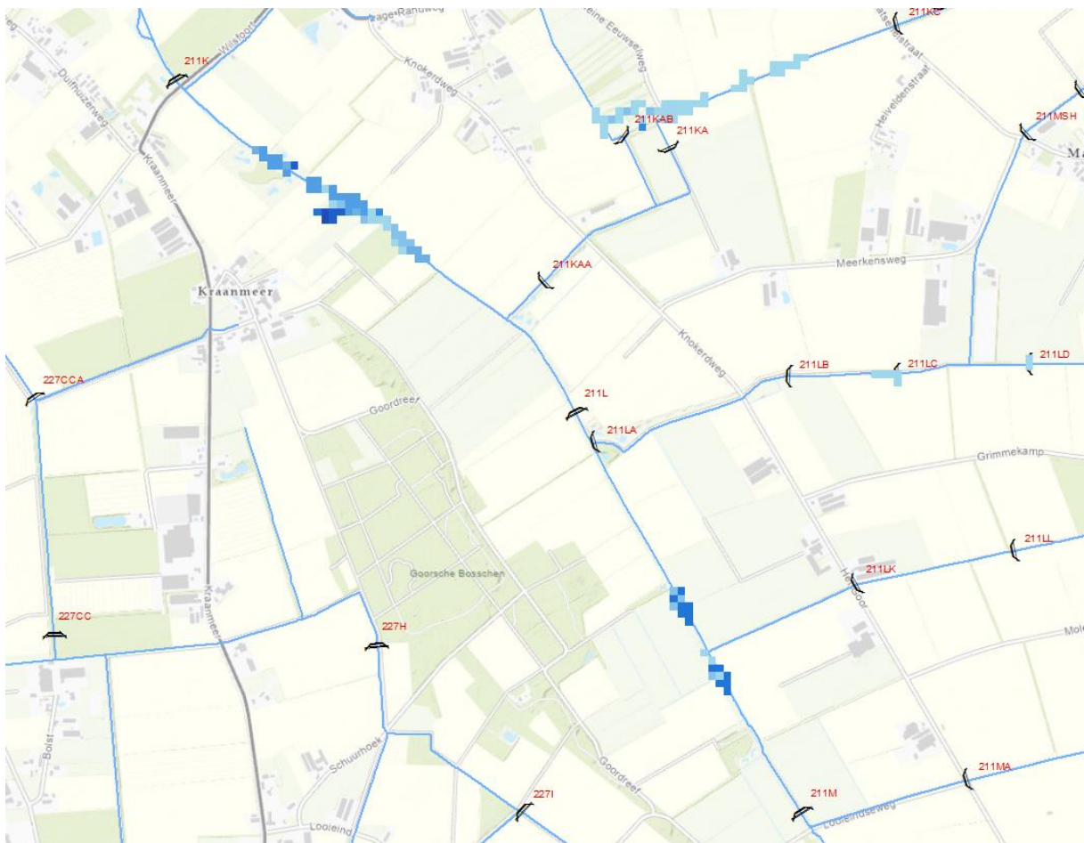
Figuur 1, inundatiekaart huidige situatie
