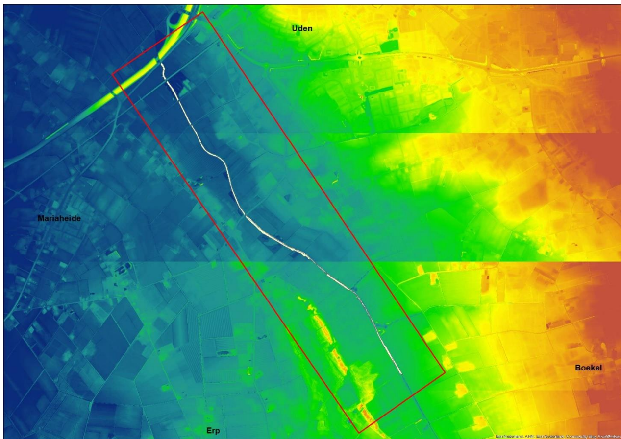
Figuur 3 Actueel Hoogtebestand Nederland Leijgraaf traject A50 (Bron: Esri Nederland)
