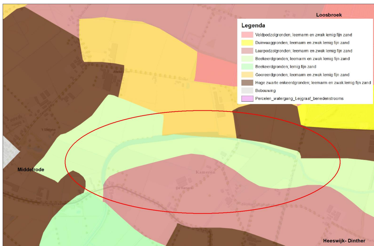
Figuur 7 Bodemkaart Leijgraaf Middelrode (Bron: Esri Nederland)
