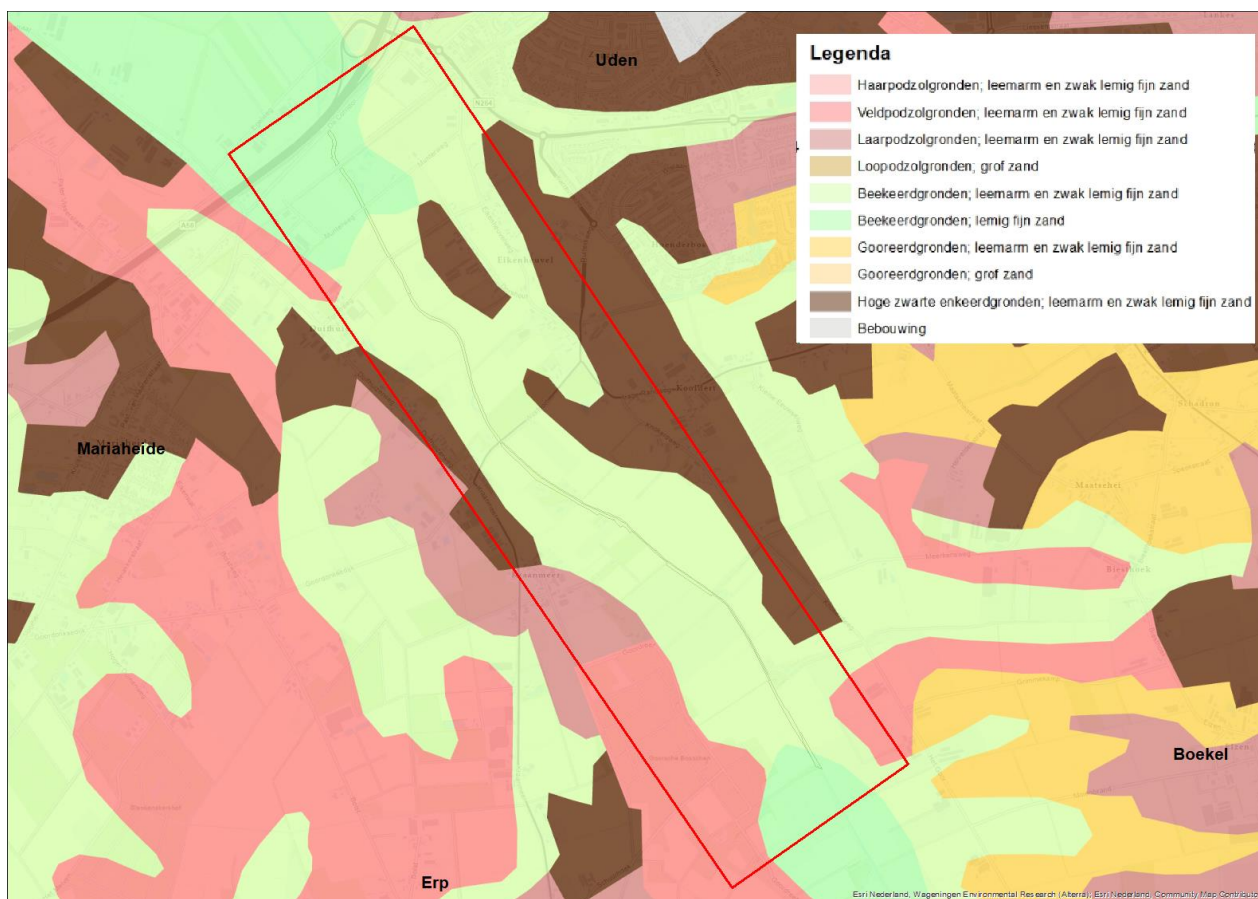
Figuur 8 Bodemkaart Leijgraaf A50 (Bron: Esri Nederland)
