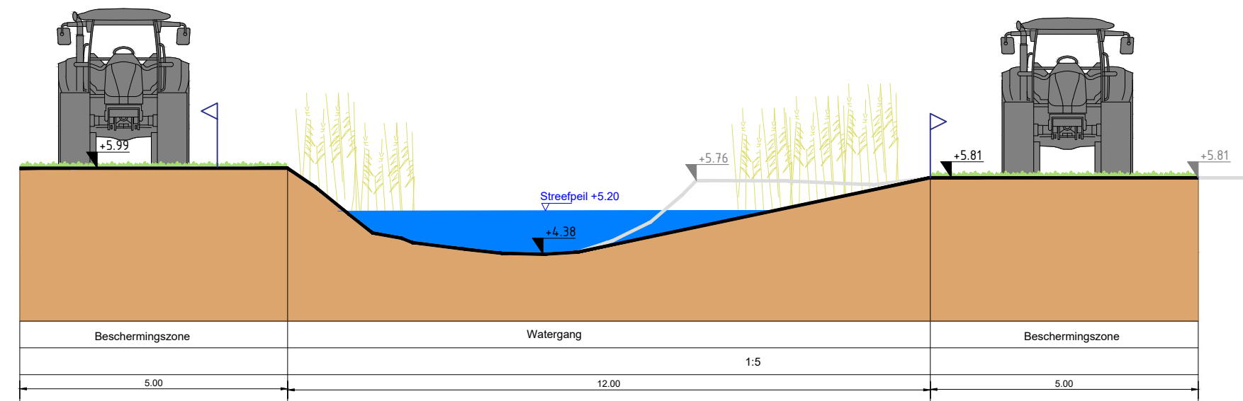
Profiel D-D'
