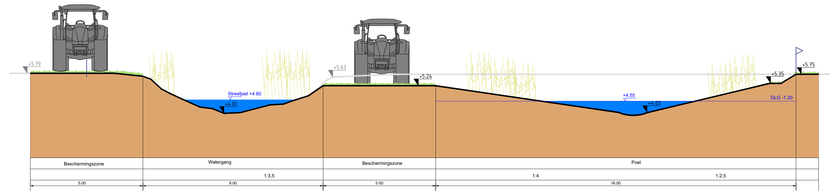
Profiel C-C'
