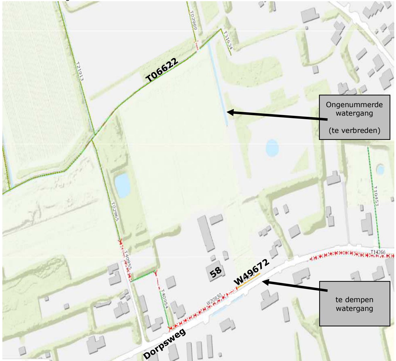
Overzichtstekening
