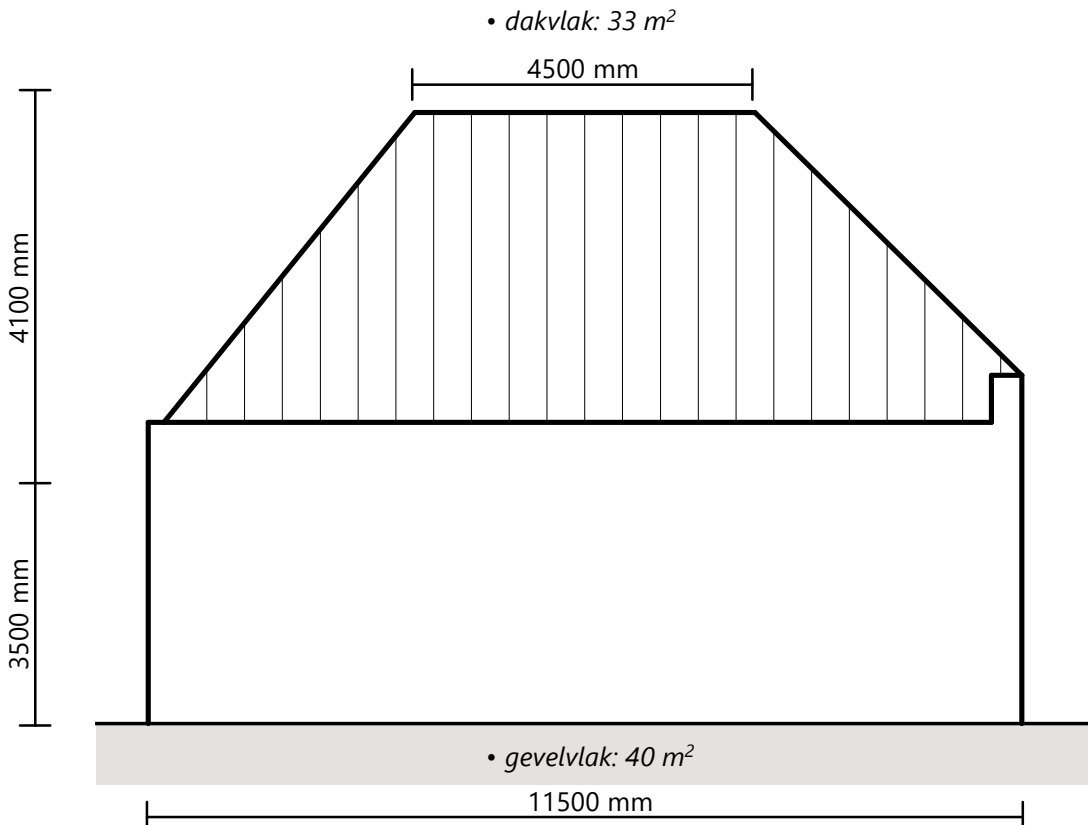
LINKERGEVEL
