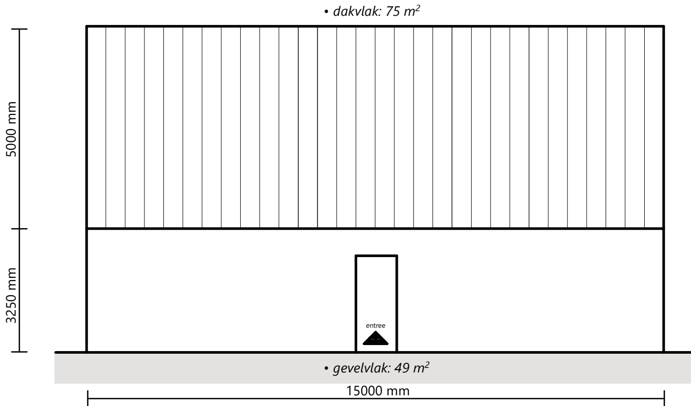
VOORGEVEL
