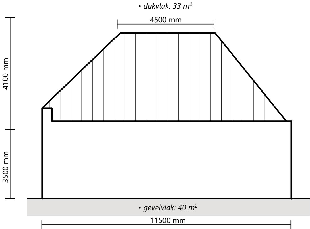
RECHTERGEVEL
