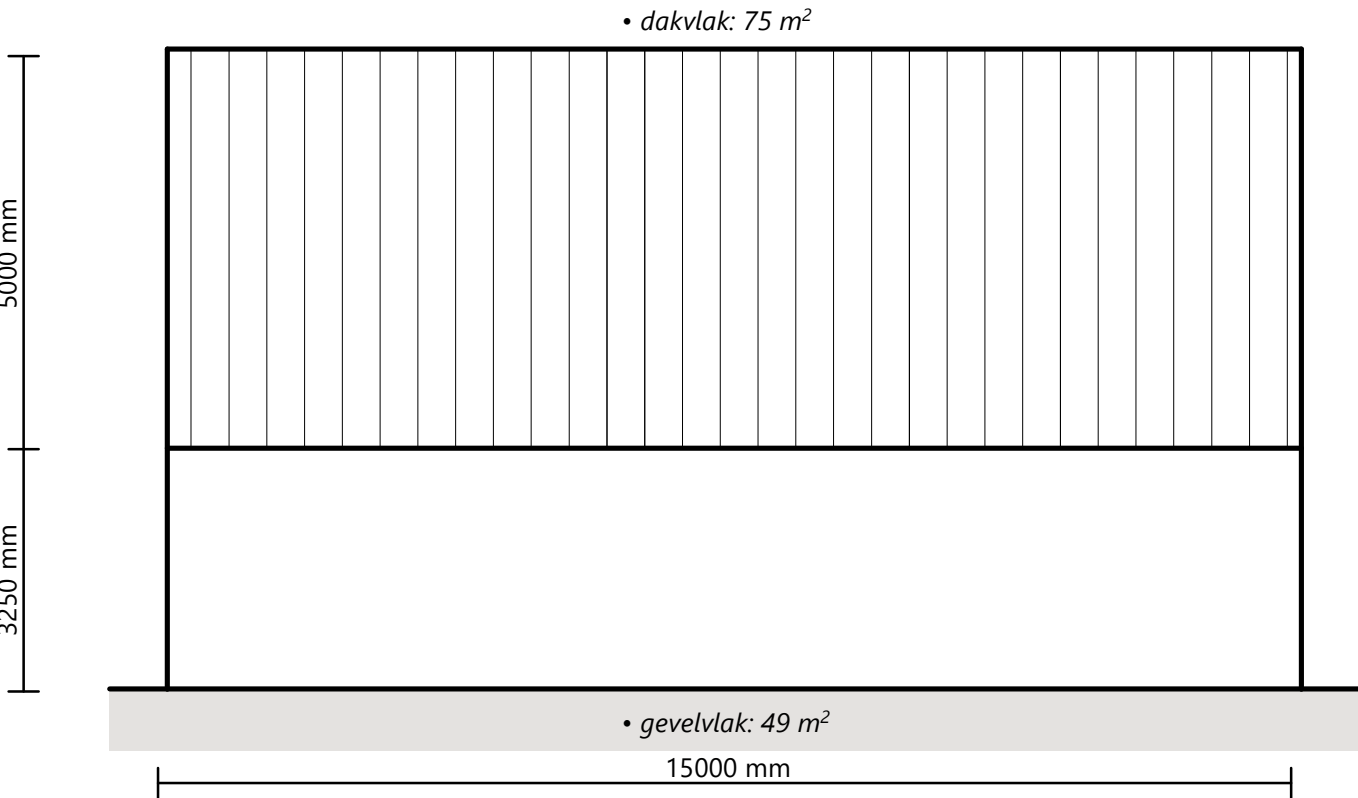
ACHTERGEVEL
