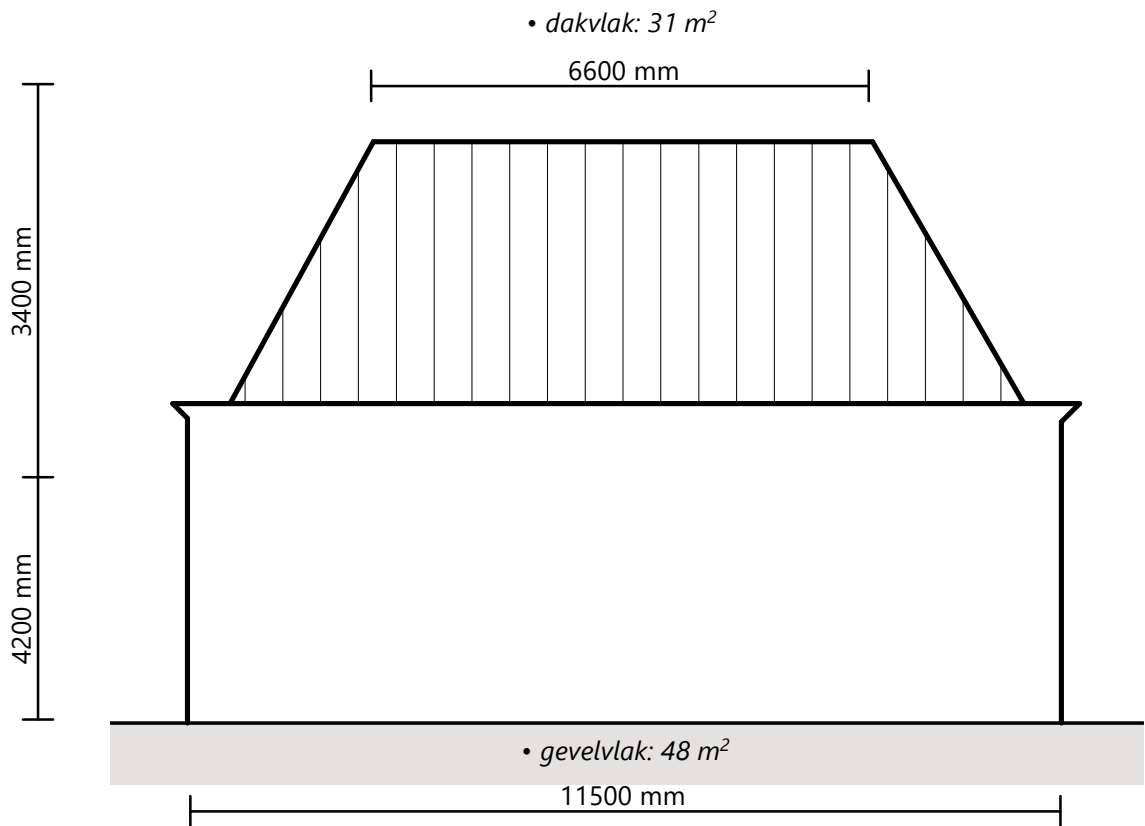
VOORGEVEL
