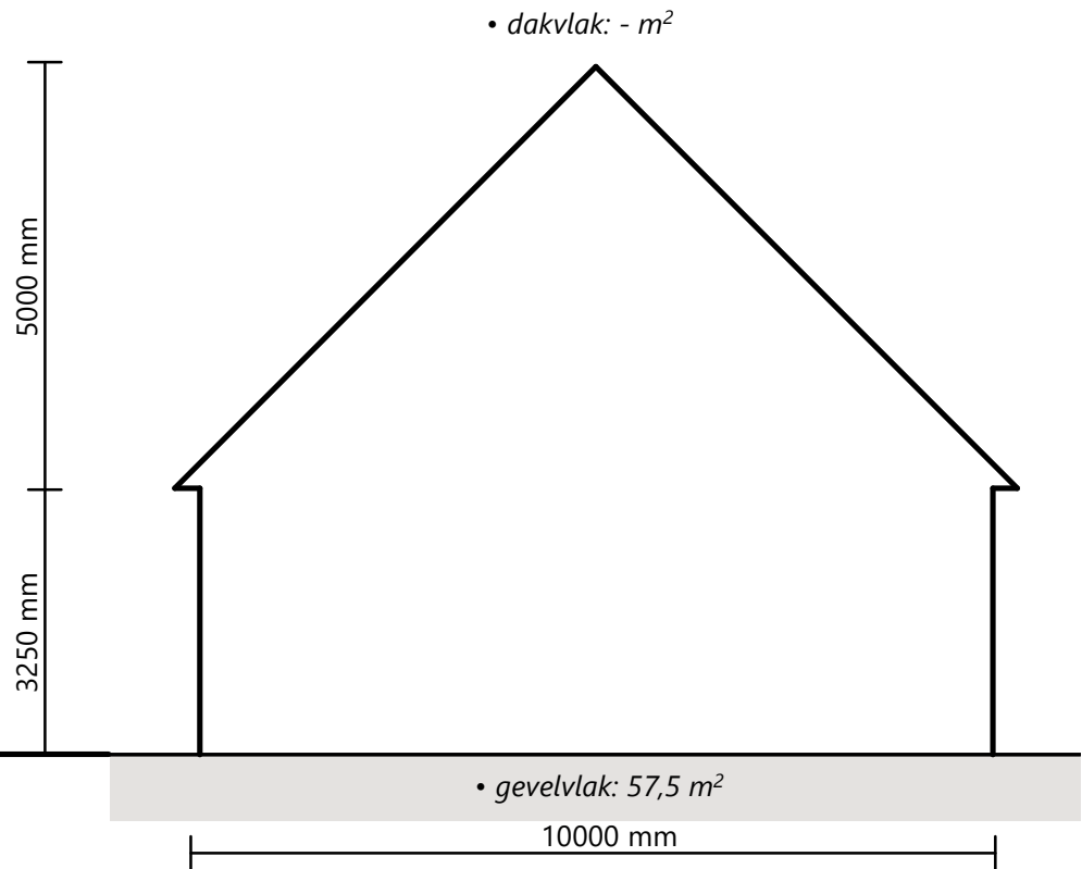
RECHTERGEVEL
