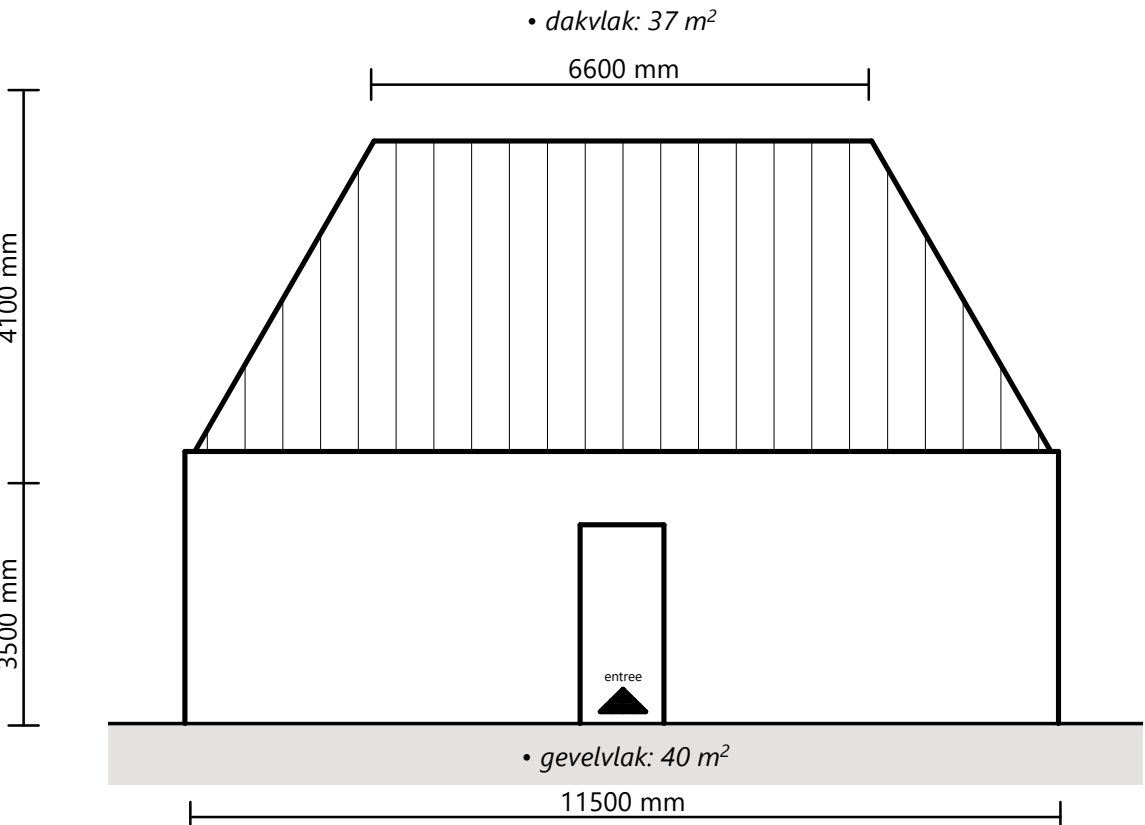
ACHTERGEVEL
