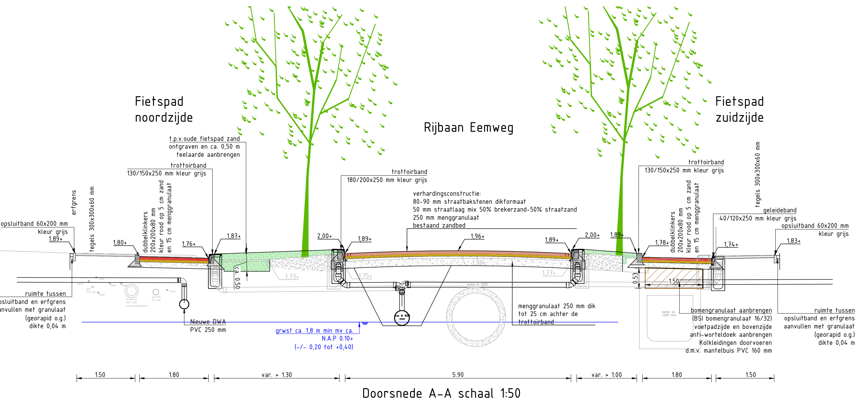
Doorsnede A-A schaal 1:50
