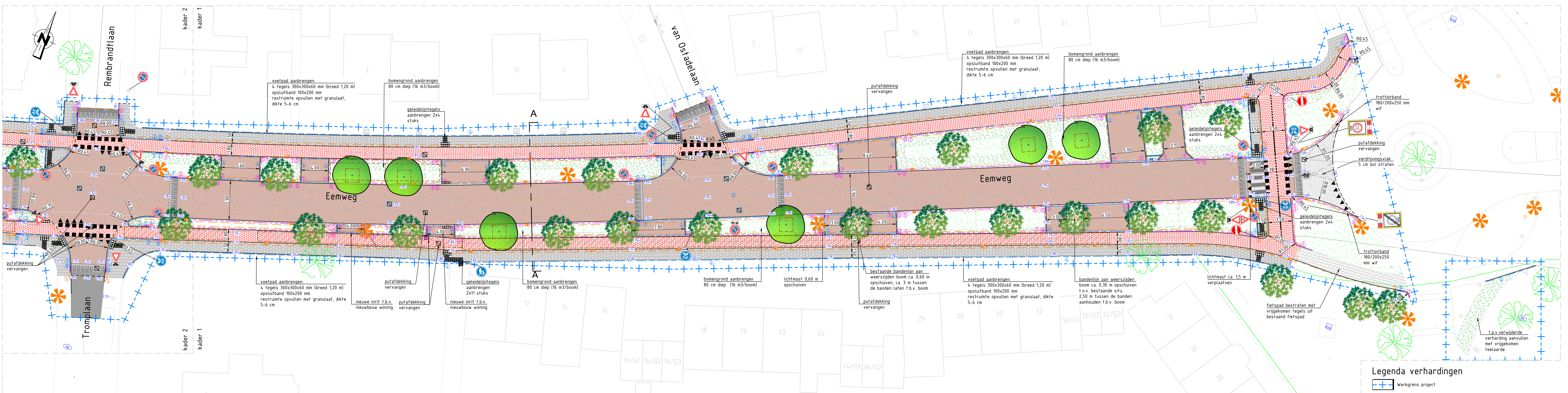
Bovenaanzicht opruimen en aanbrengen riolering deel oost (kader 1 schaal 1:200)
