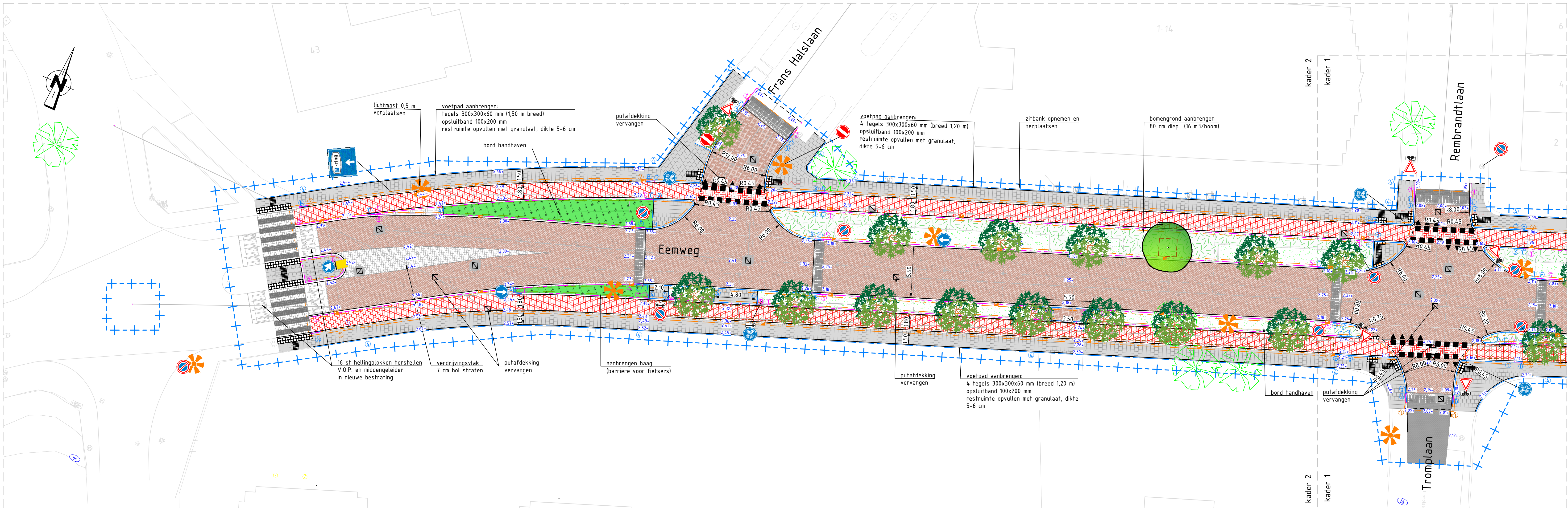
Bovenaanzicht opruimen en aanbrengen riolering deel west (kader 2 schaal 1:200)
