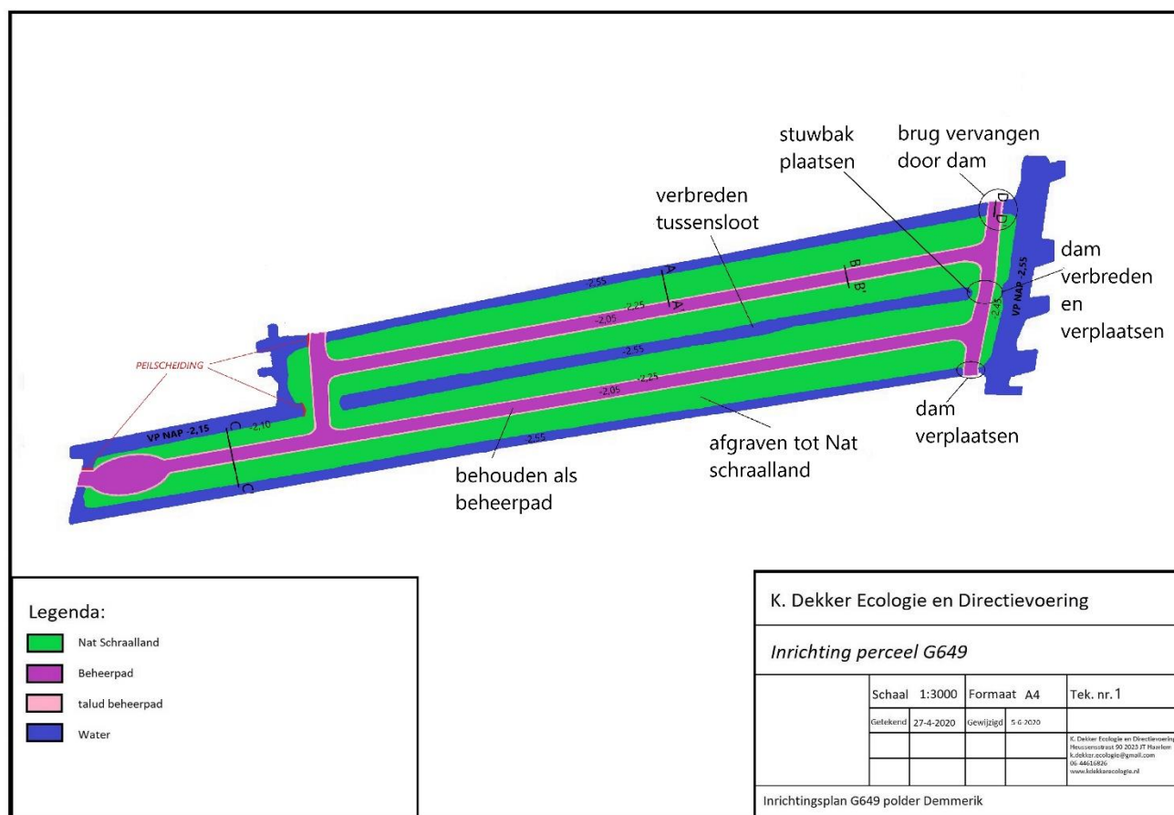
Figuur 3 kaart inrichtingsplan met locatie van te plaatsen stuw.
