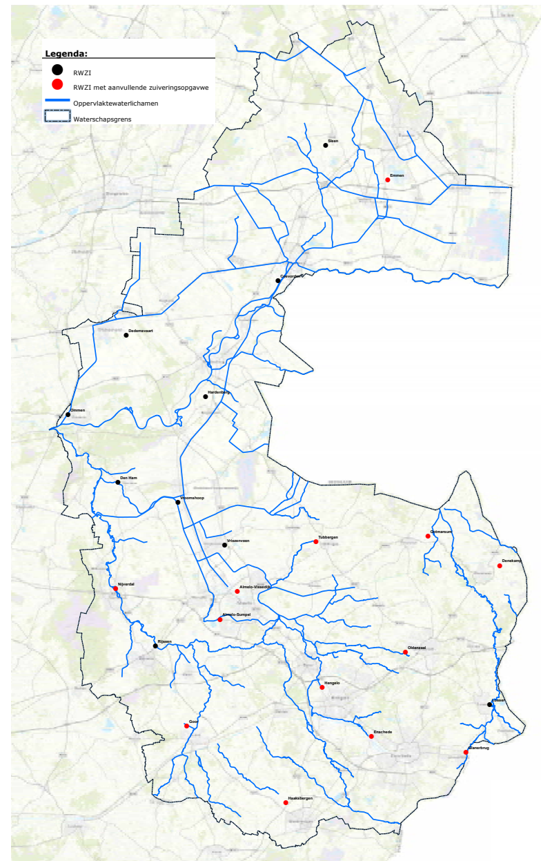
Figuur 4-2. Te verbeteren rwzi's (rode punten) vanuit doelbereik KRW.
