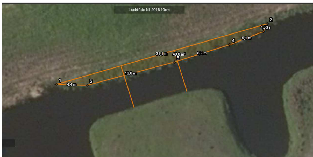
Figuur 2 - graven 40 m 2 door over recht te 'trekken'. Nieuwe breedte op de waterlijn wordt 6 meter
