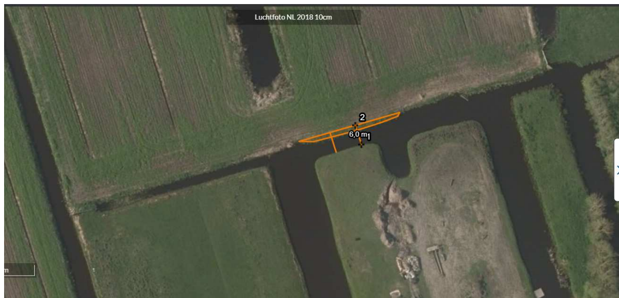
Figuur 2 - graven 40 m 2 door over recht te 'trekken'. Nieuwe breedte op de waterlijn wordt 6 meter
