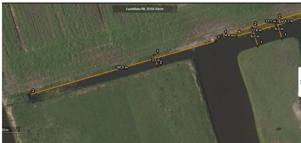
Figuur 3 - Verbreden sloot met 1 meter naar een nieuwe breedte van 3.5 m – op de waterlijn- over een lengte van 60 meter. Is 60m 2 compensatie.
