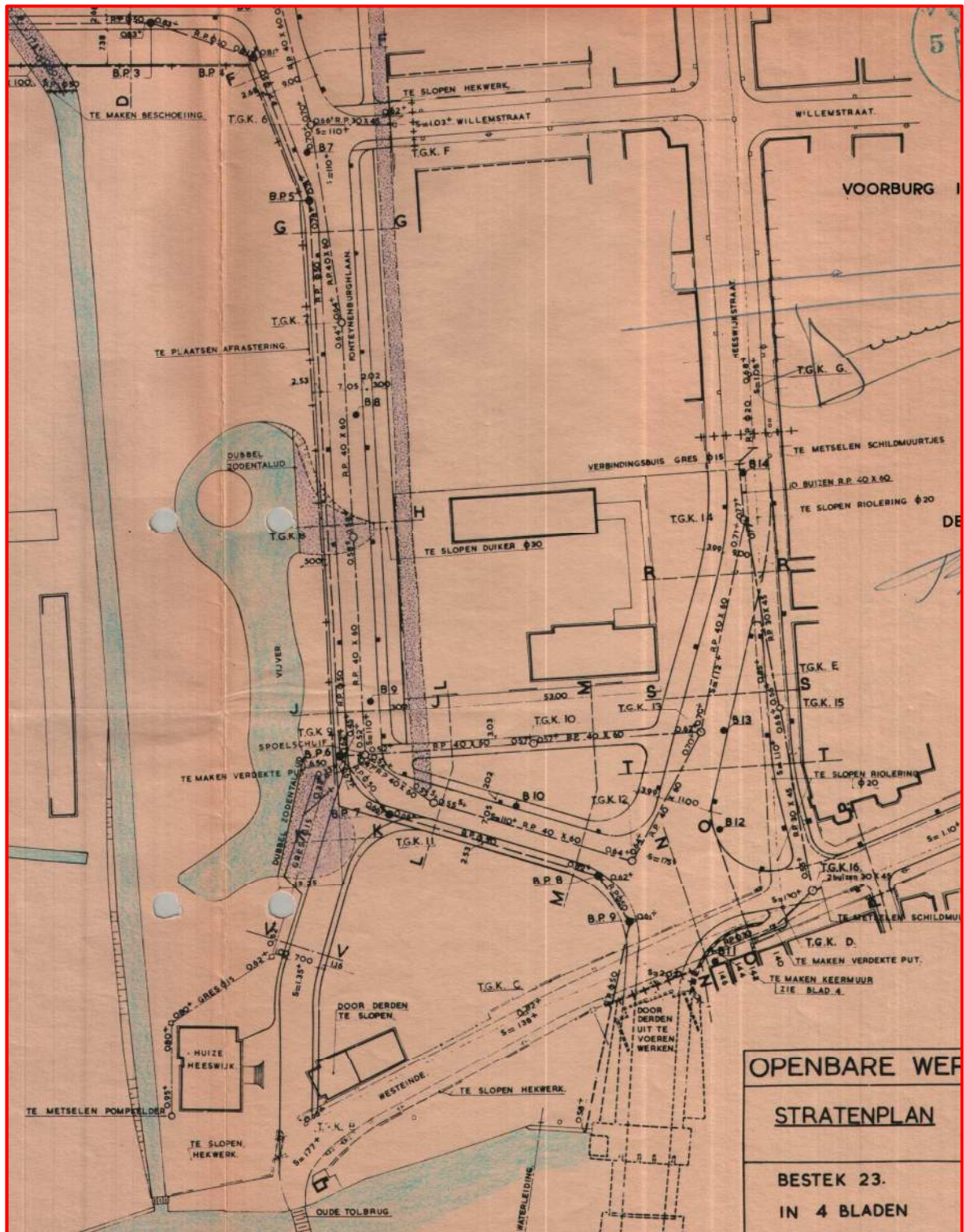
Tekening A-784; Stratenplan Heeswijk bestek 23 - 1955
