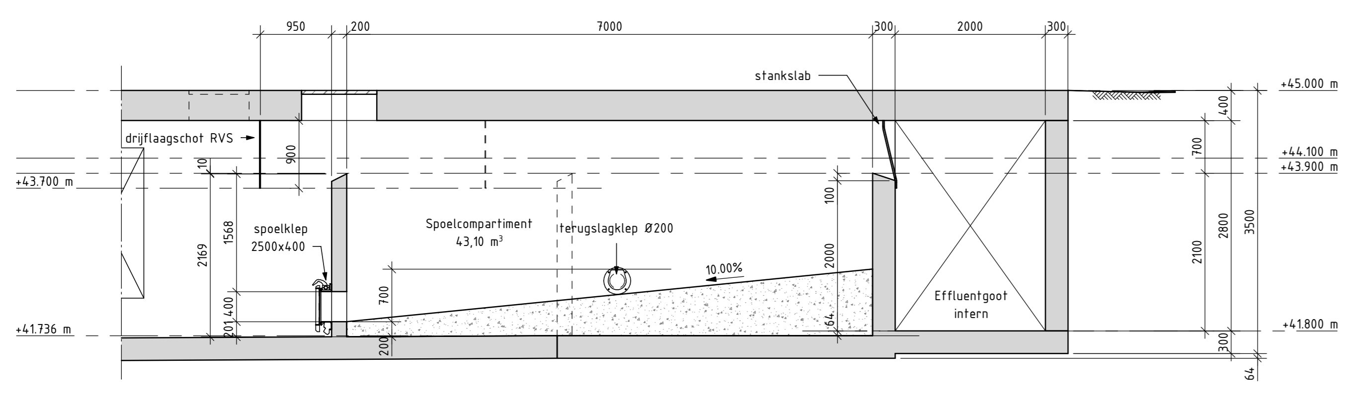
Dsn. C-C SCHAAL: 1 : 50
