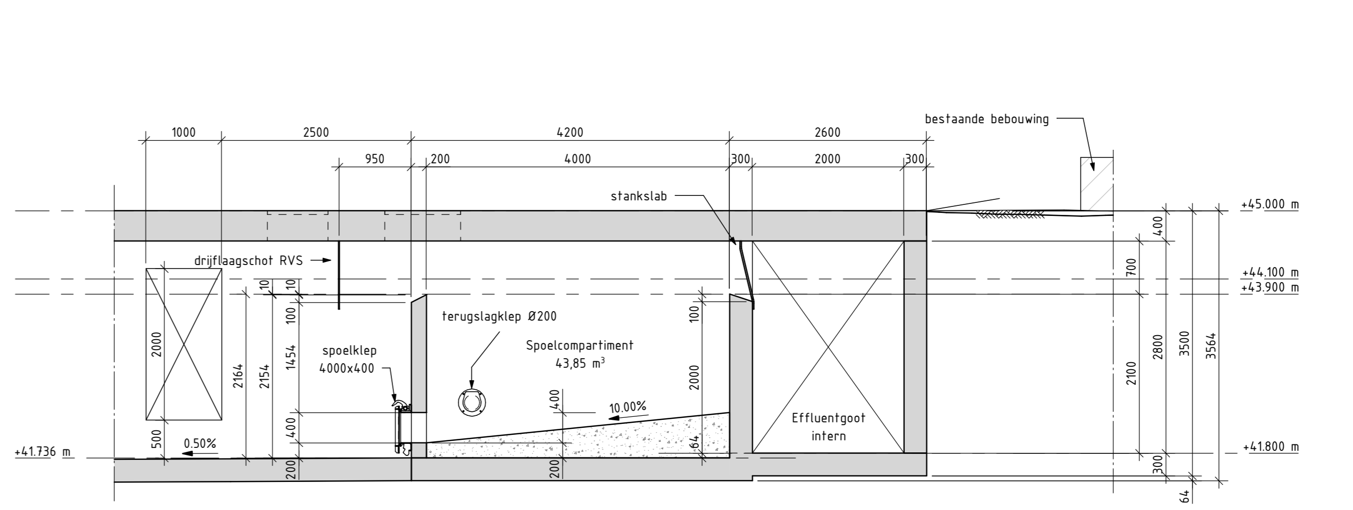
Dsn. B-B - detail 2
