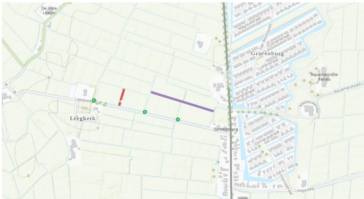
Figuur 1: Locatie van werkzaamheden. De Rode lijn geeft de te dempen watergang weer. De paarse lijn geeft de te verbreden watergang weer. De groene cirkels geven de locatie weer van de aan te leggen duikers.
