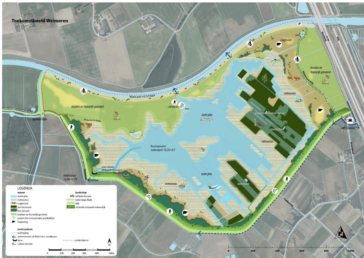
Figuur 1.2 a: Toekomstbeeld natte natuurgebied Weimeren, inclusief robuuste natuurkering
