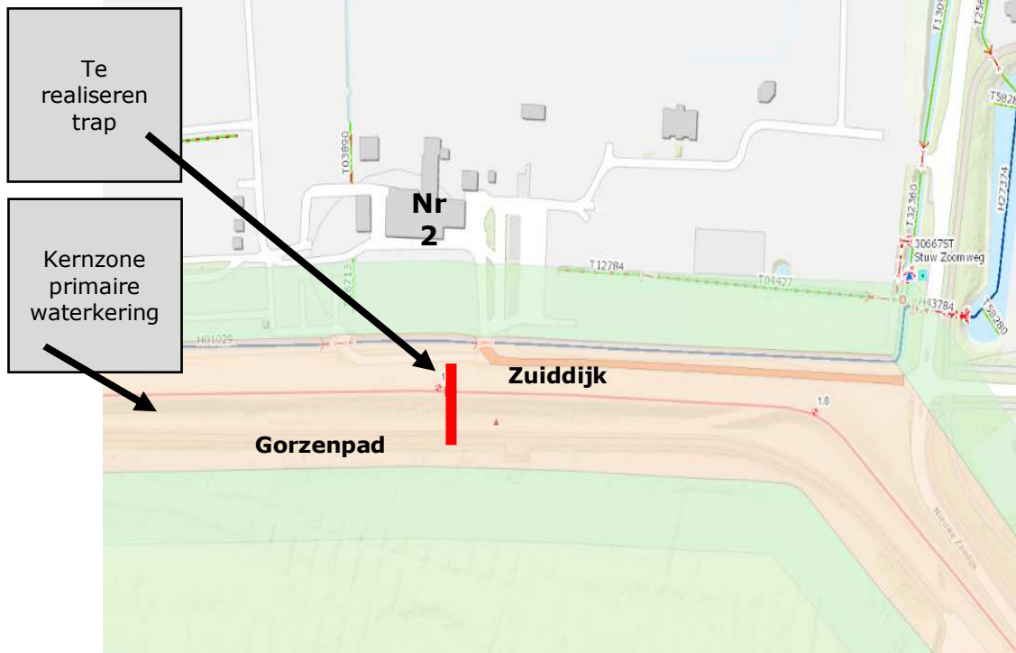
Detailtekening 2
