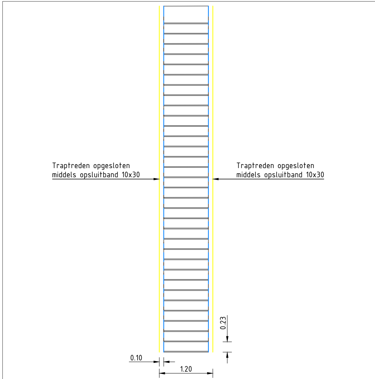
Bovenaanzicht trap
