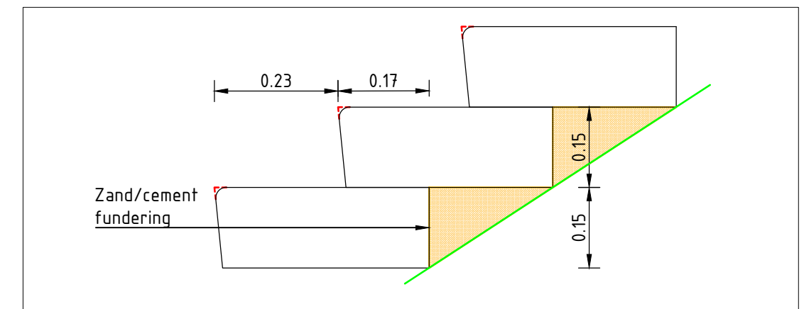
Uitvoering traptreden
