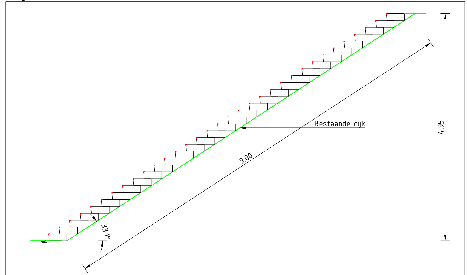
Zijaanzicht trap
