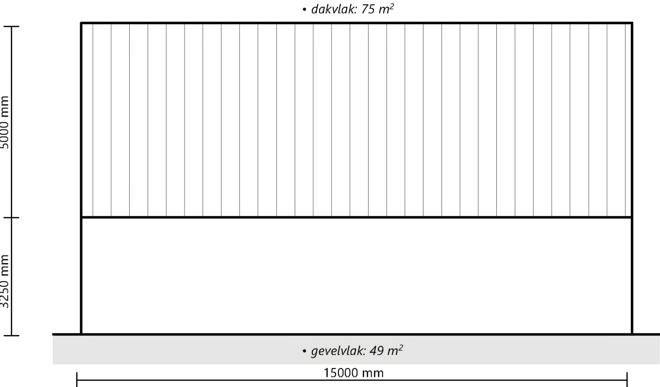
ACHTERGEVEL
