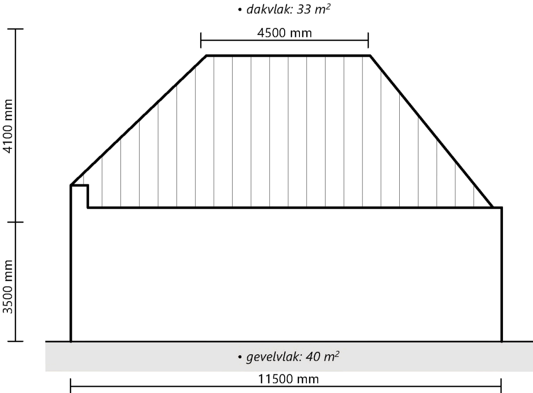
RECHTERGEVEL
