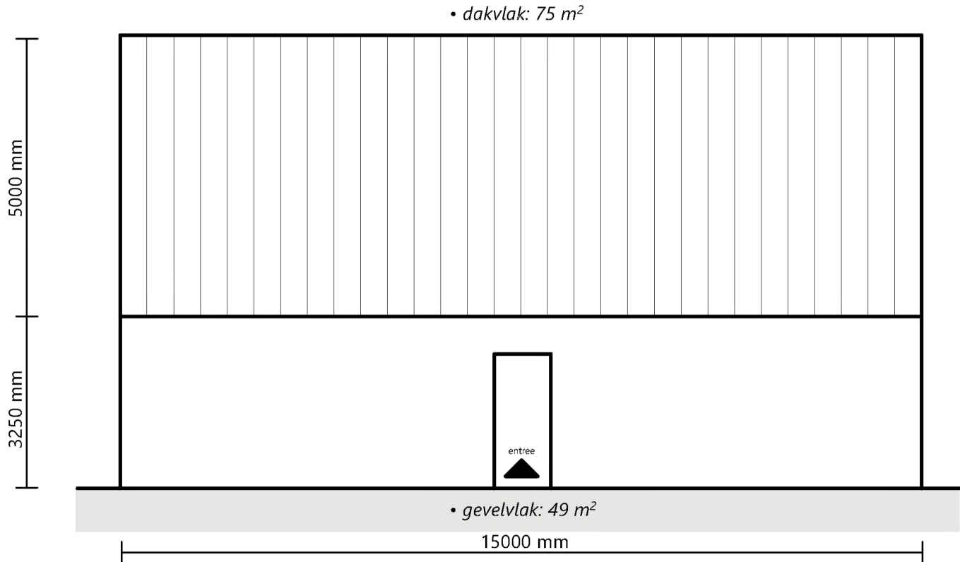
VOORGEVEL
