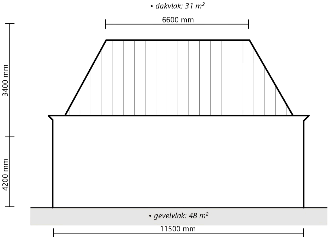
VOORGEVEL
