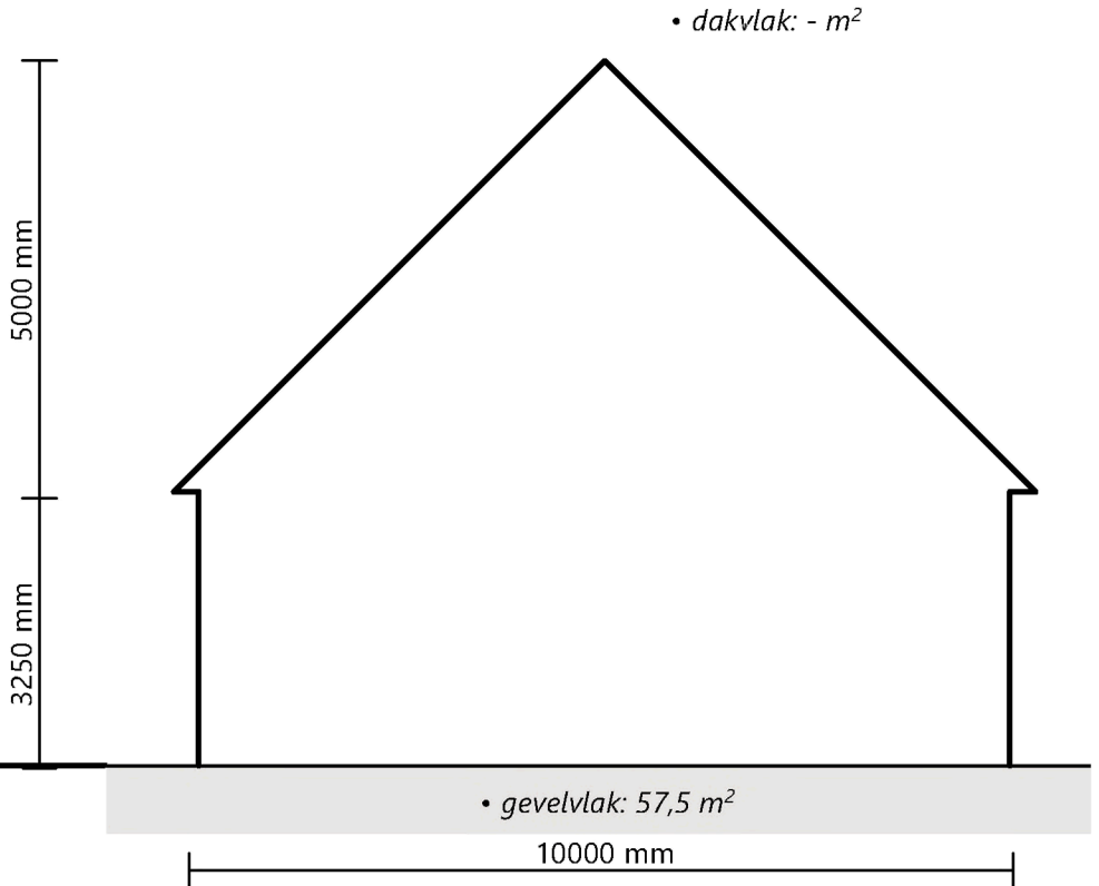
LINKERGEVEL
