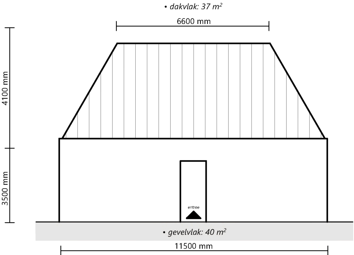
ACHTERGEVEL
