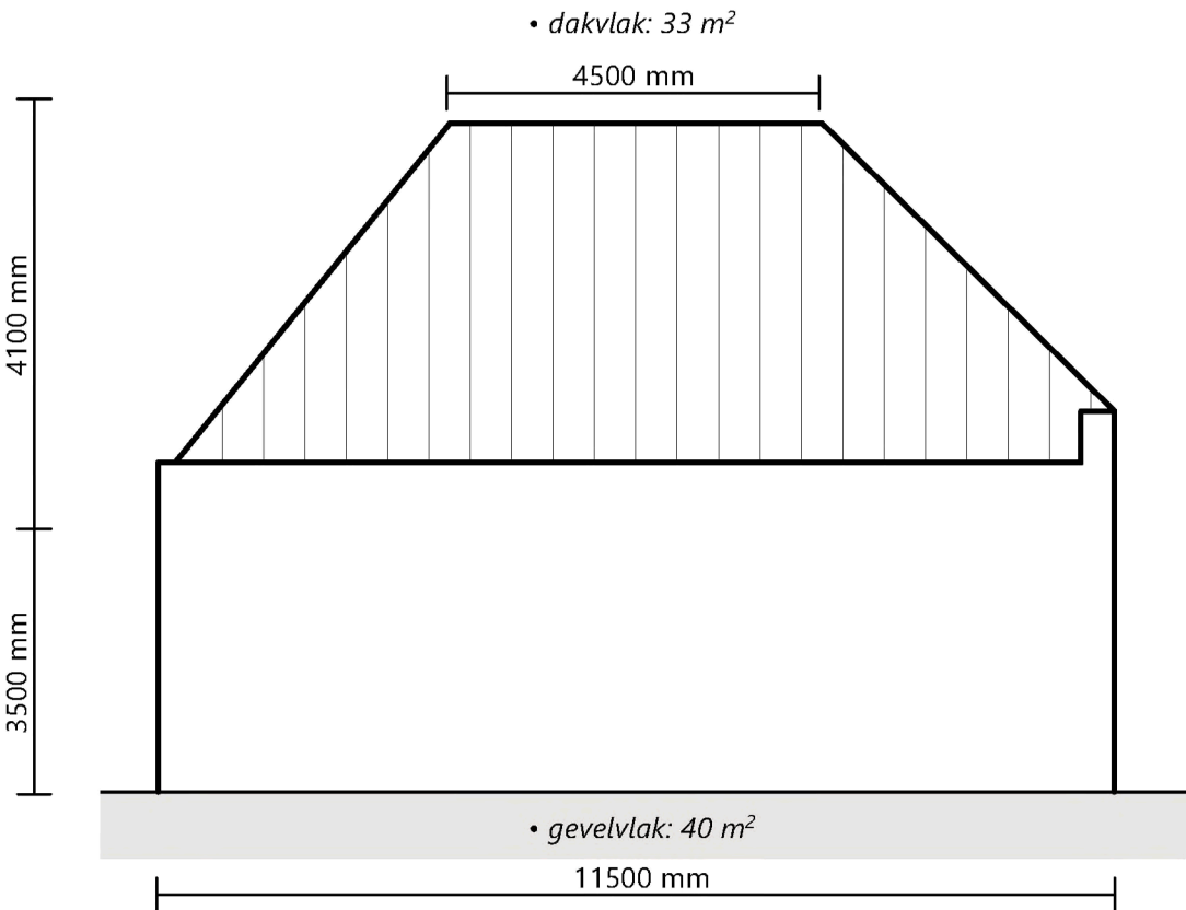
LINKERGEVEL
