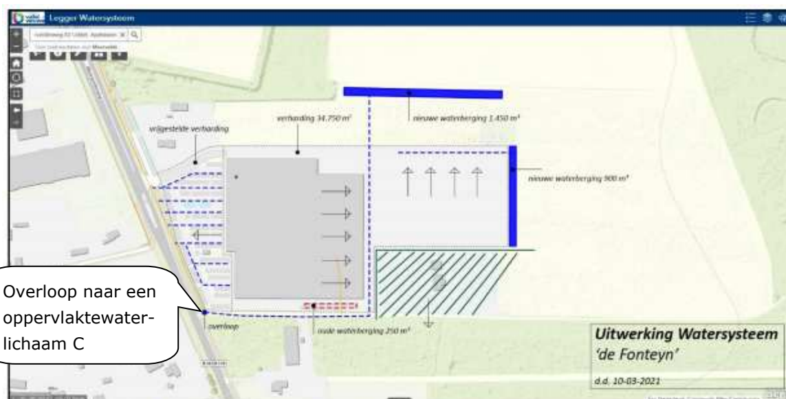
Figuur 1, Schematische weergave watersysteem Meervelderweg 52 – Uddel.
