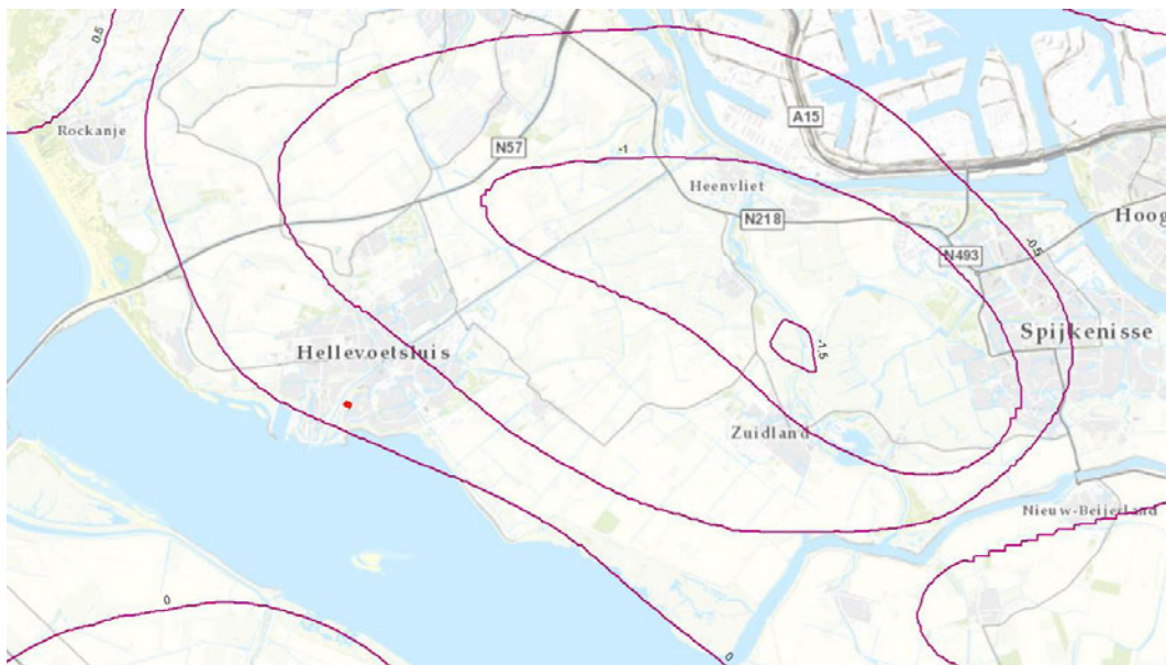
Figuur 2.13: Isohypsens grondwater Eerste Watervoerend Pakket
