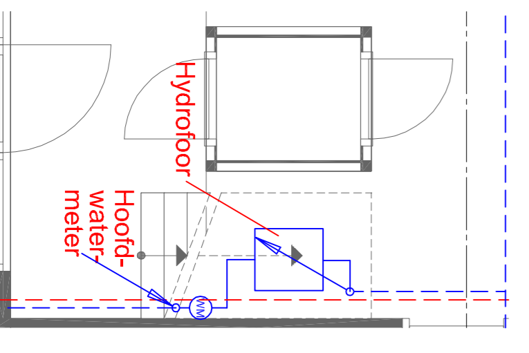
Detail hydrofoor, schaal 1:50
