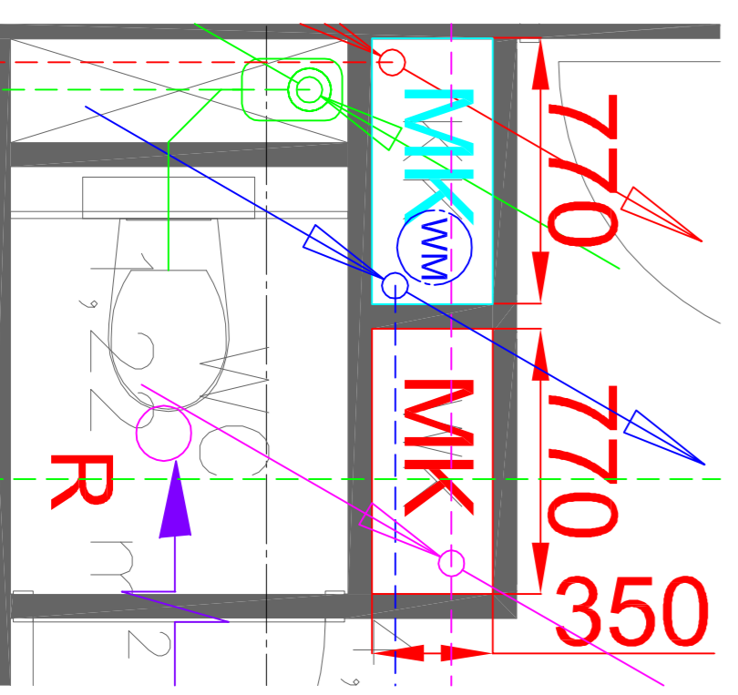
Detail entreegebied, schaal 1:20
