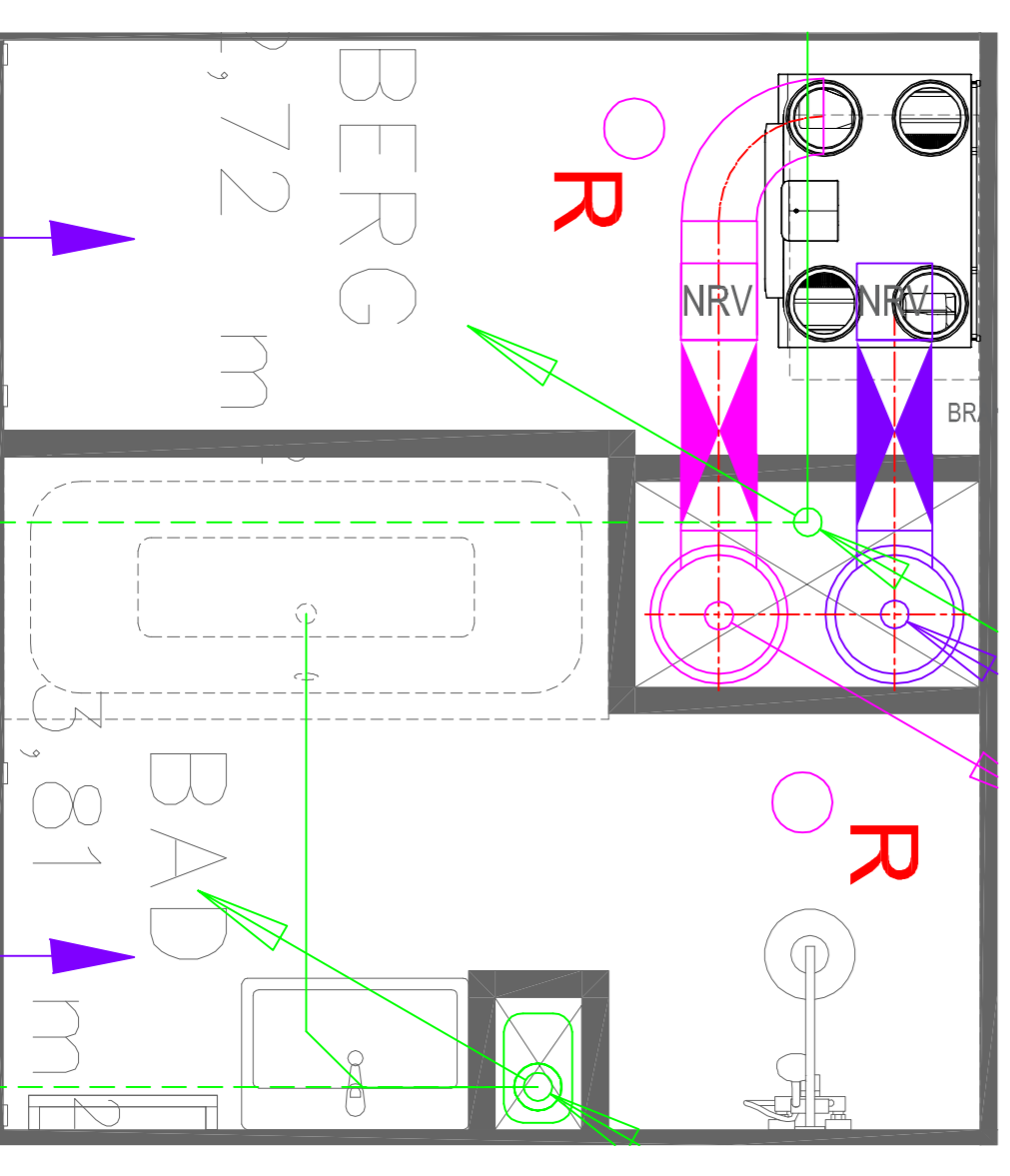
Detail berging / TR schaal 1:20 (zie tevens tekening W-301)
