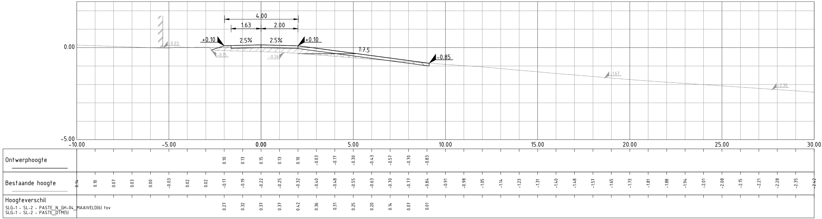
DWP-36.1 Schaal 1:100
