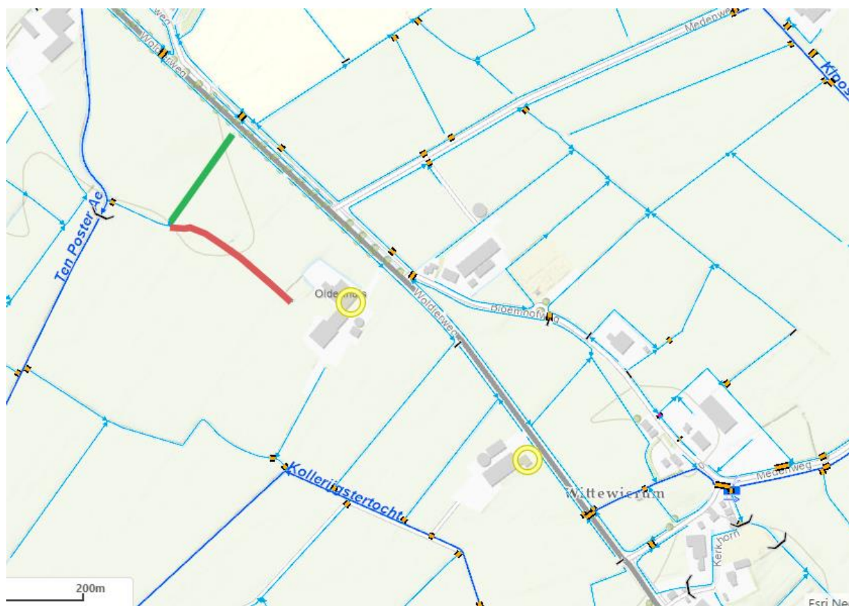
Figuur 1: Bovenstaand figuur geeft globaal het werkgebied weer. De rode lijn geeft de te dempen watergang weer, de groene lijn geeft de te verbreden watergang weer.
