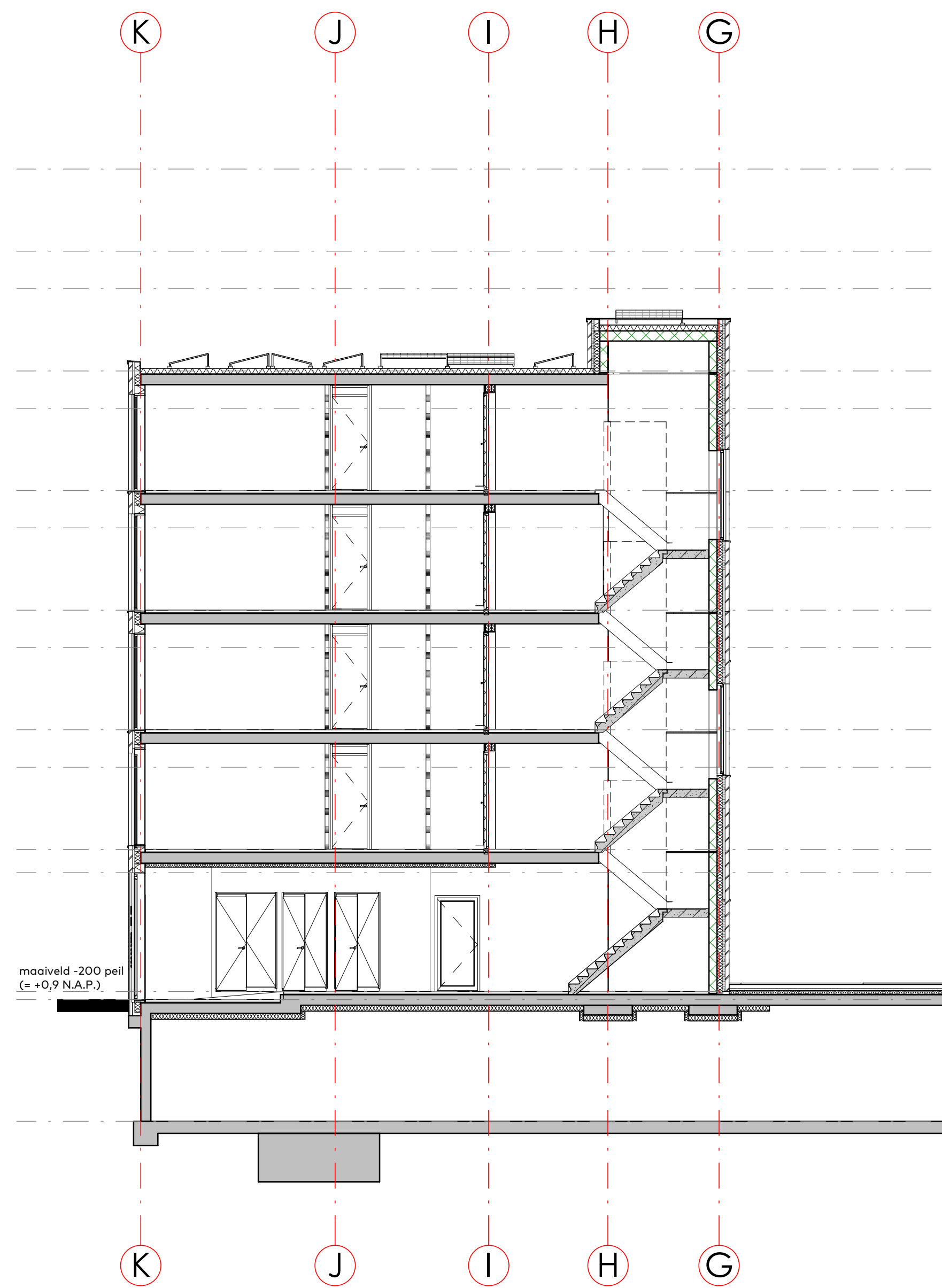
Doorsnede E
