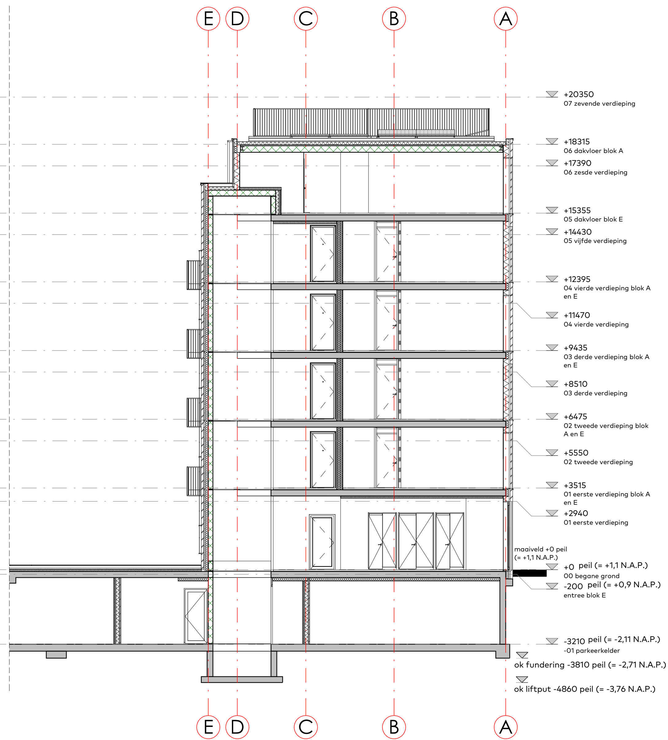
Doorsnede E'
