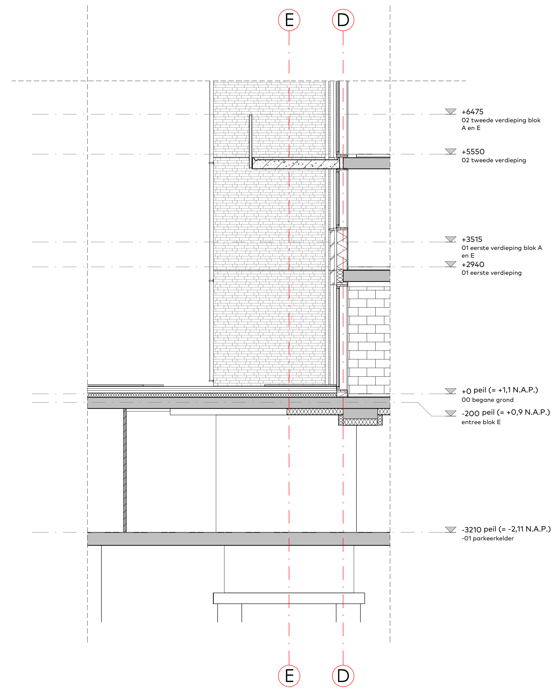
Doorsnede F' (1:50)
