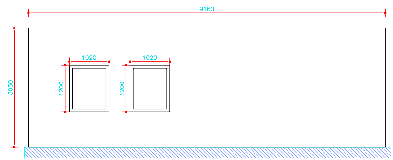
Aanzicht 2
