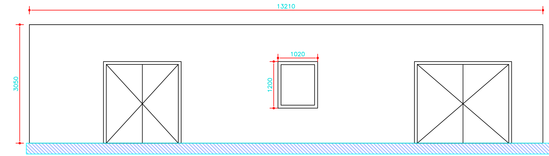
Aanzicht 3
