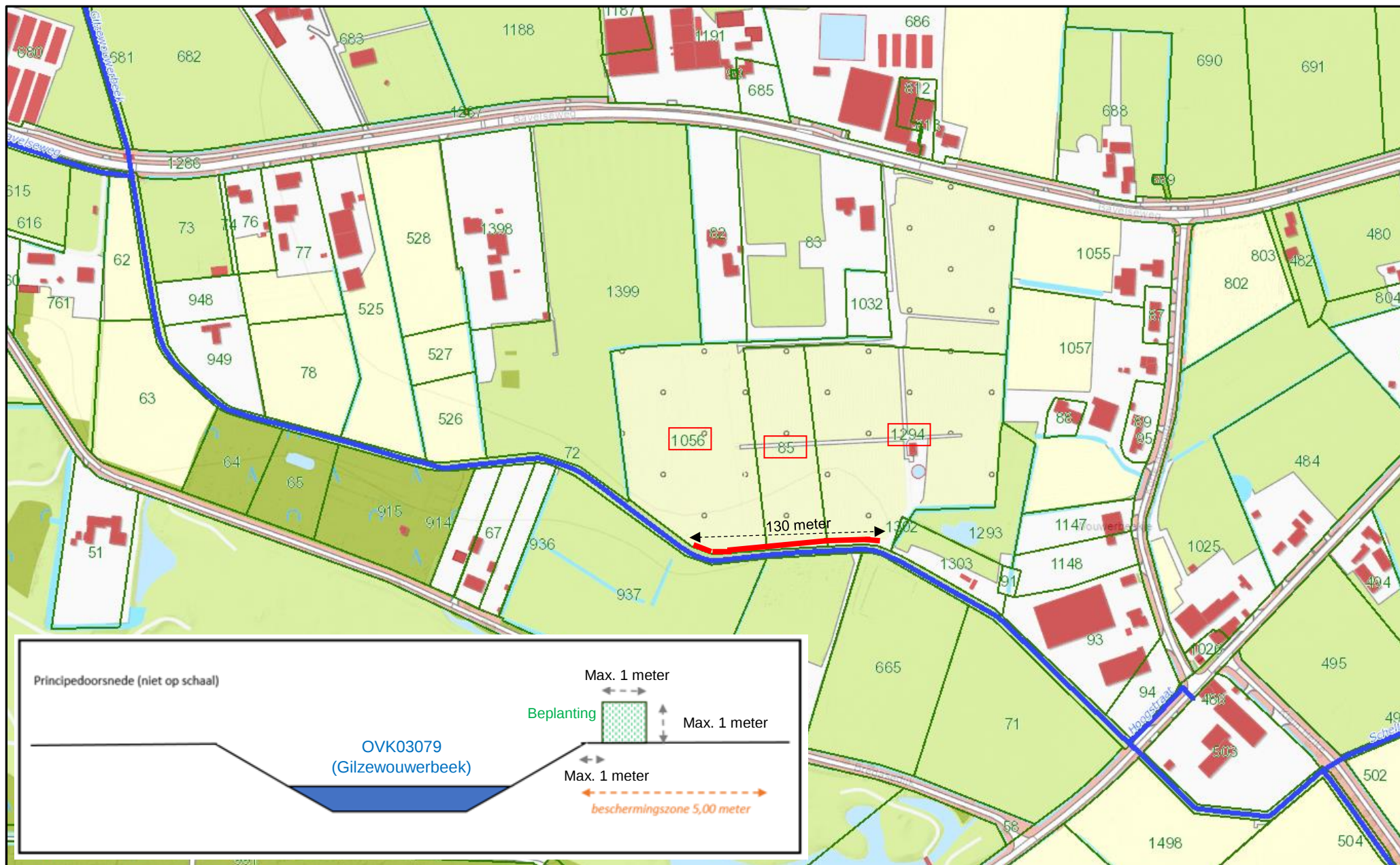
390509-B Kadastrale situatie
