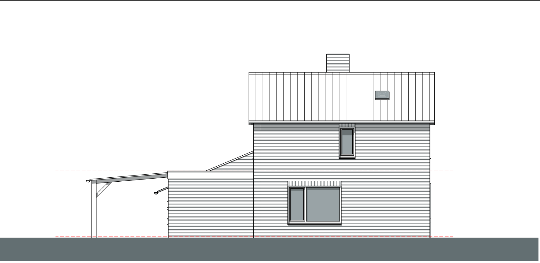
linker zijgevel
