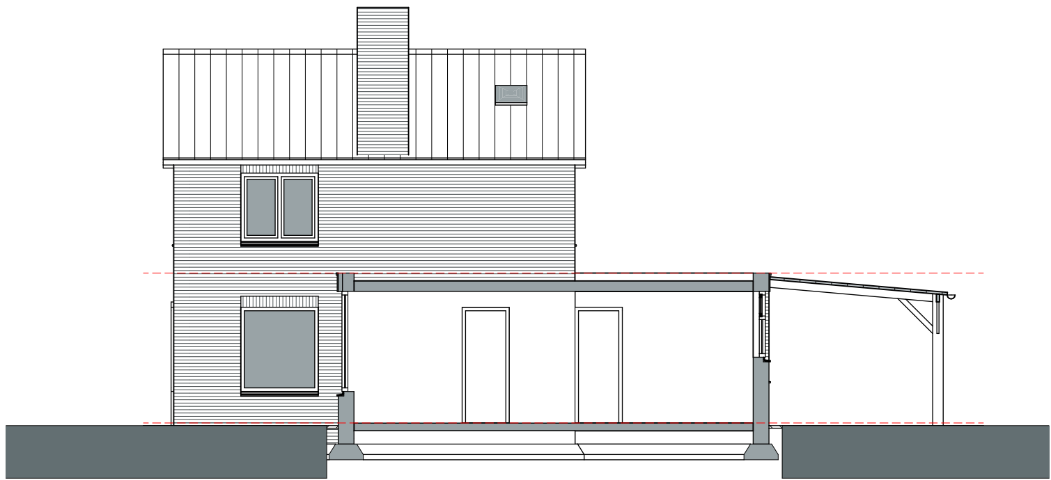
doorsnede C-C rechter zijgevel woning
