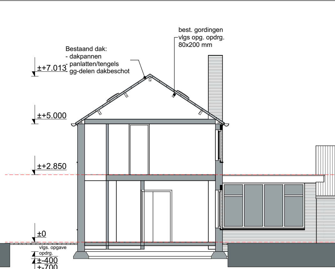
doorsnede A-A
