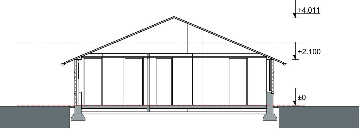
doorsnede B-B
