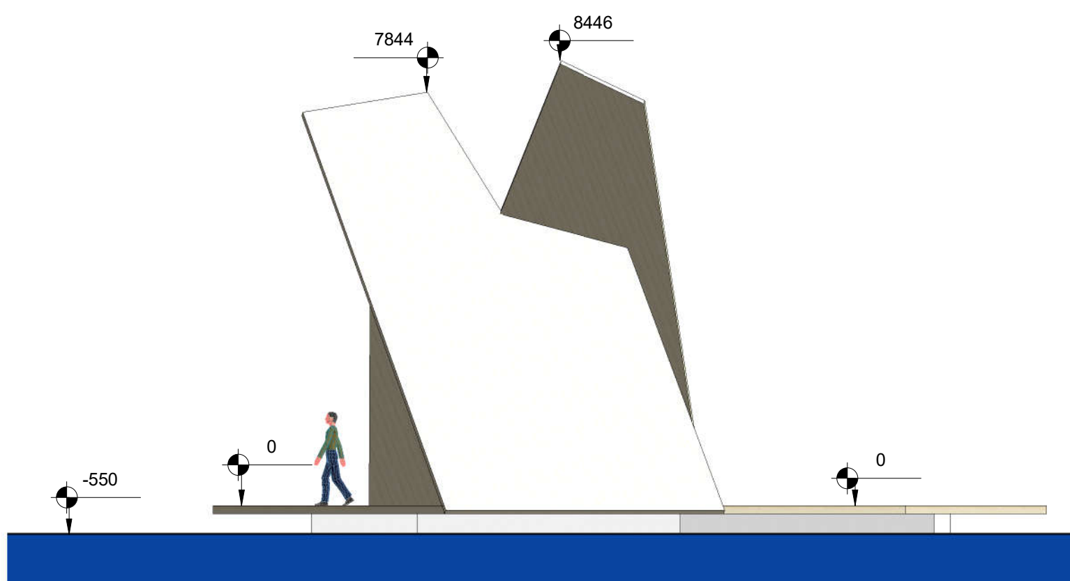
2 Linkerkant 1 : 100
