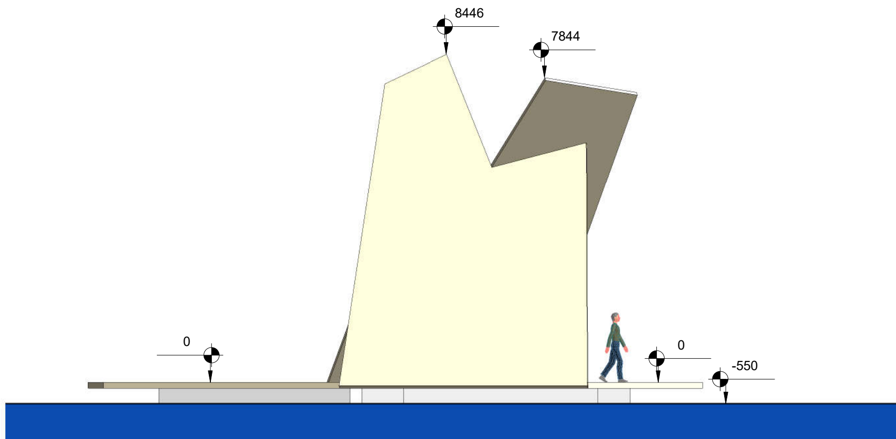
1 Rechterkant 1 : 100
