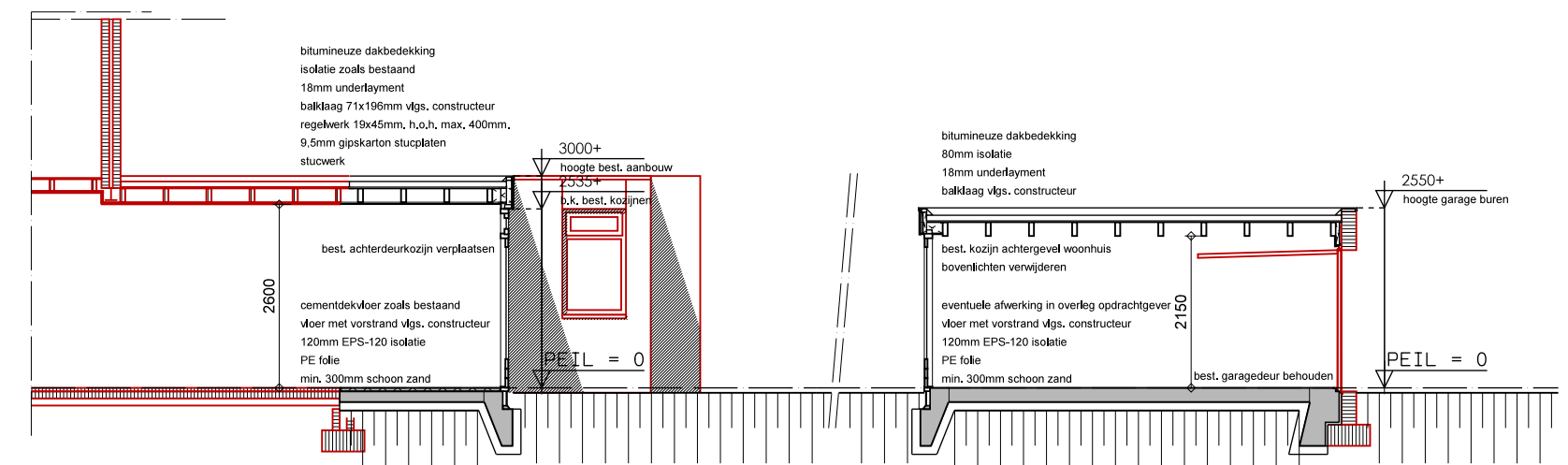
doorsnede A-A / zijaanzicht
