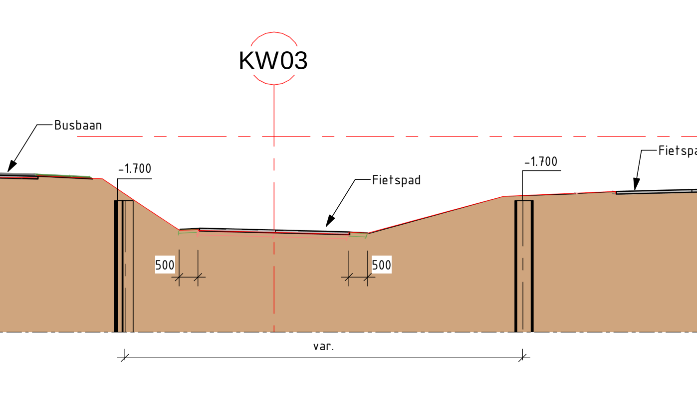
DOORSNEDE H-H schaal: 1 : 100
