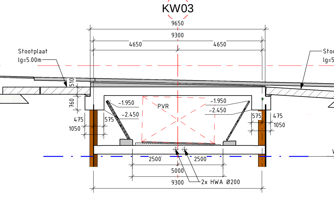
DOORSNEDE F-F schaal: 1 : 100
