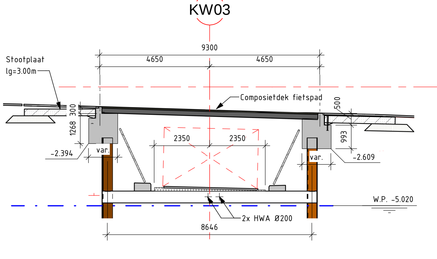
DOORSNEDE D-D schaal: 1 : 100
