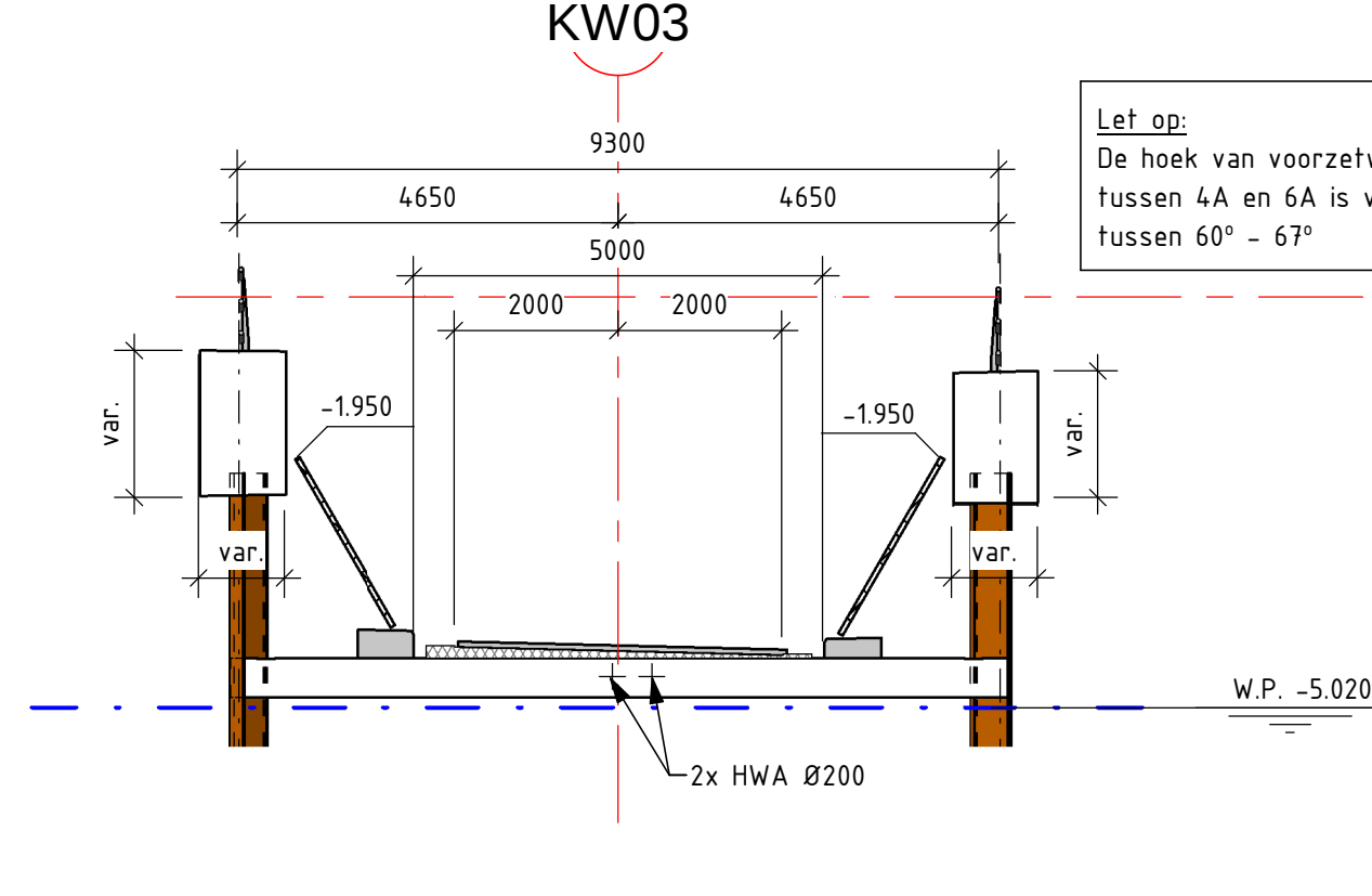
DOORSNEDE E-E schaal: 1 : 100
