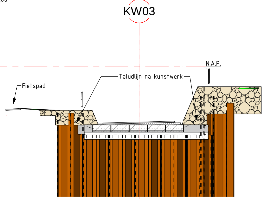
AANZICHT A-A schaal: 1 : 100
