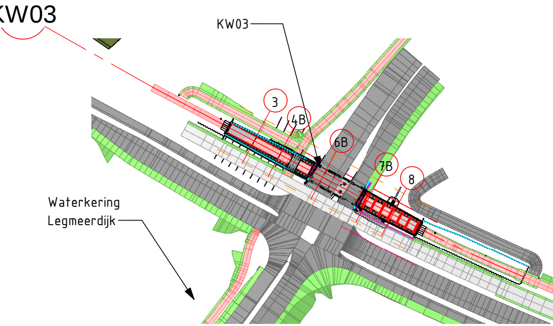
Situatie 1 : 2000
