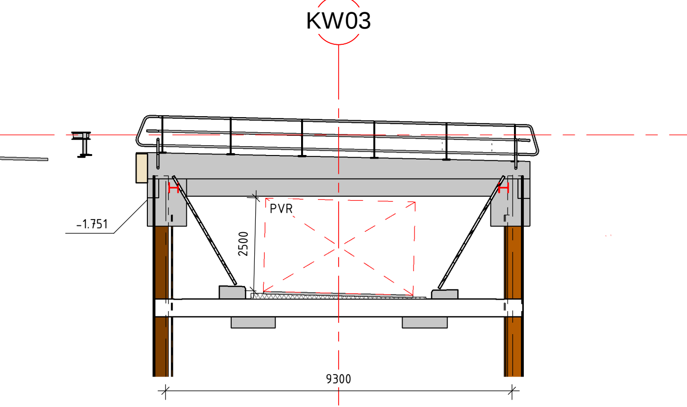
AANZICHT G-G schaal: 1 : 100
