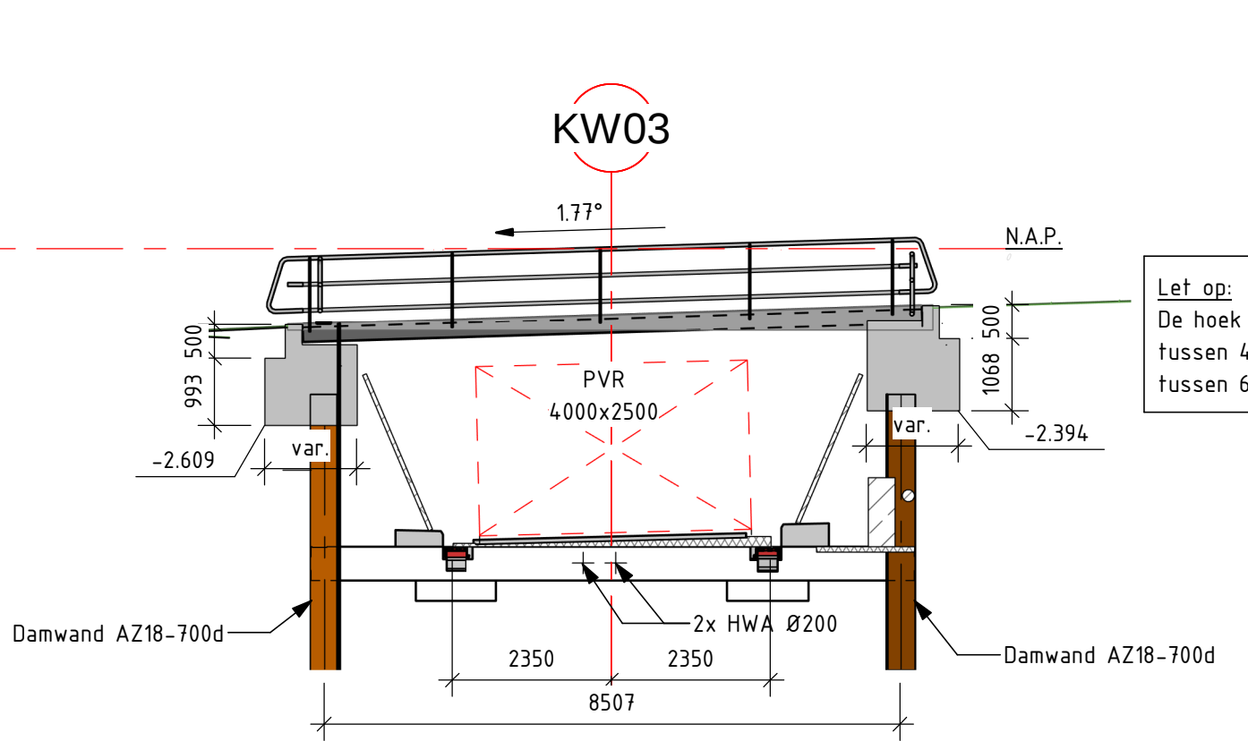
AANZICHT C-C schaal: 1 : 100
