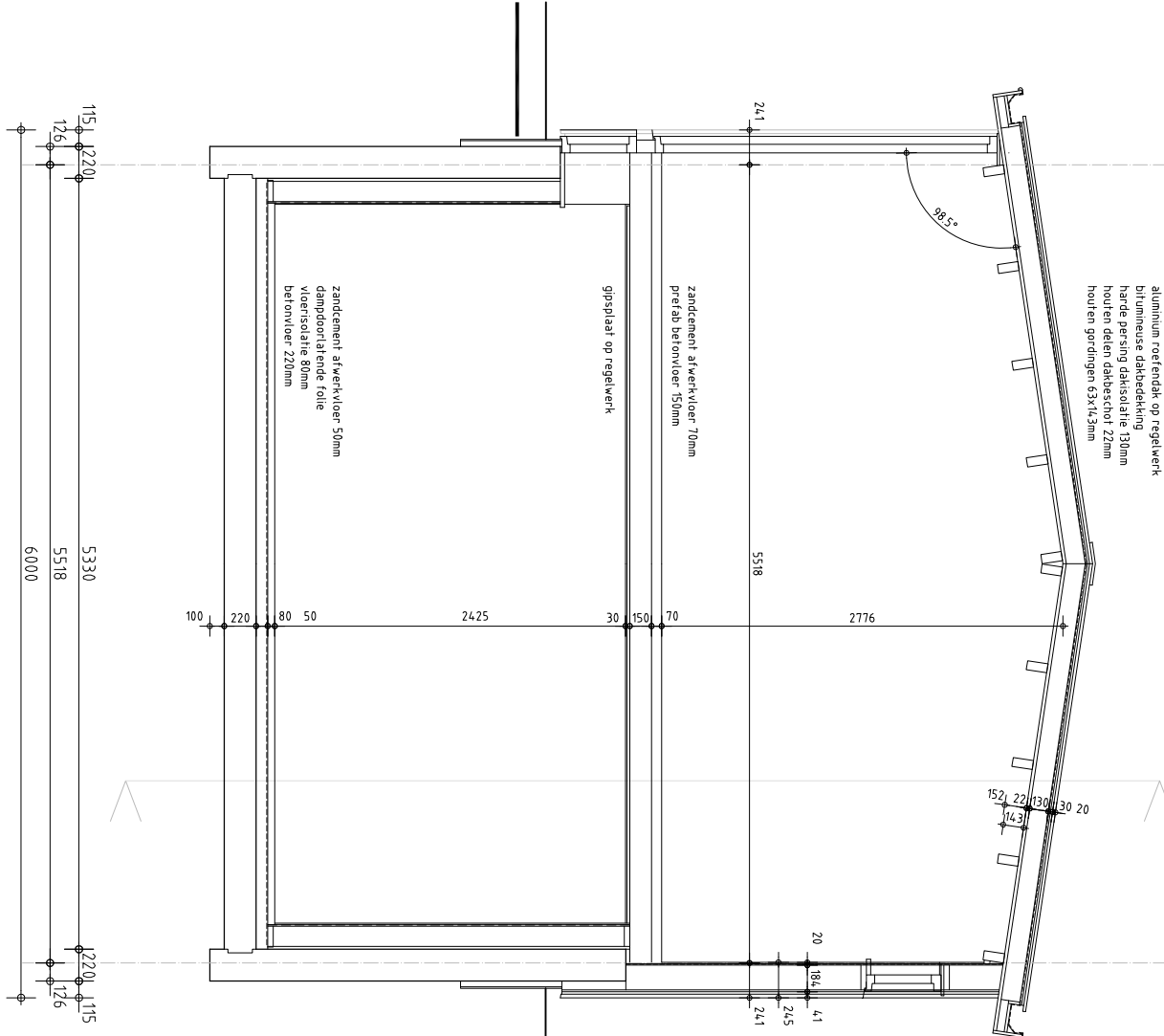
principe dwarsdoorsnede schaal 1:50
