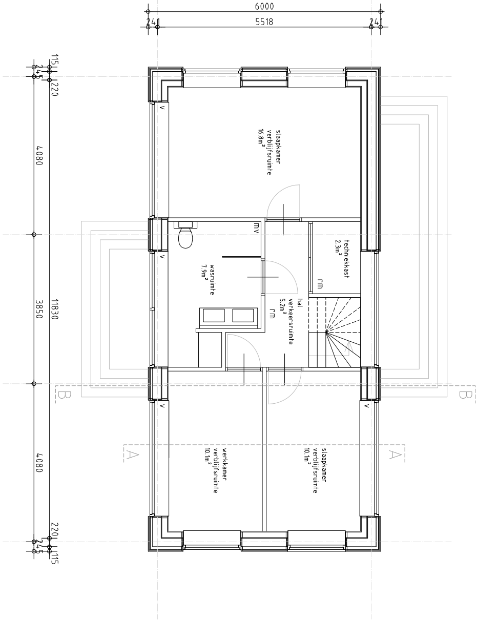
verdieping -1 schaal 1:100
