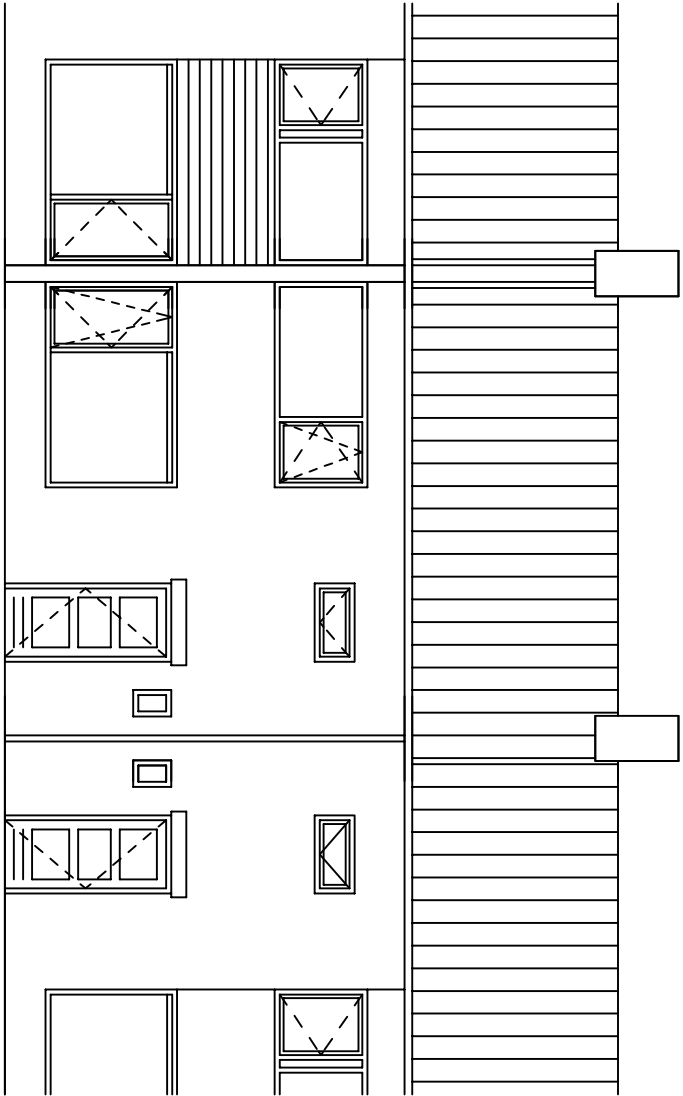
voorgevel nieuw
