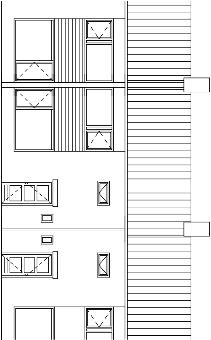
voorgevel bestaand
