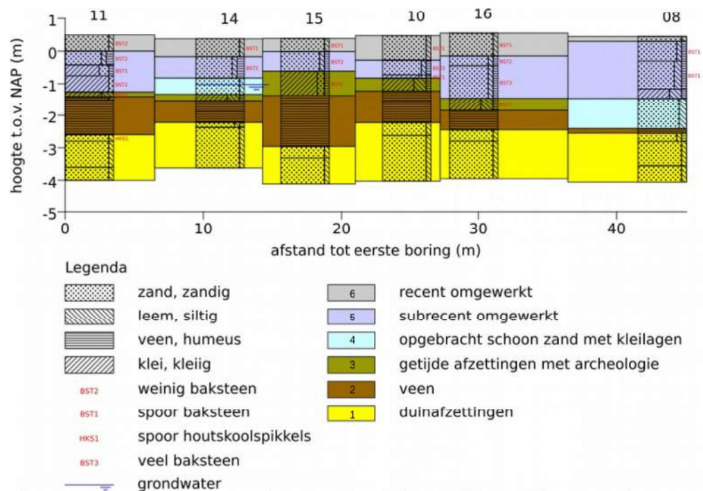
Figuur 5: Schematische doorsnede met getekende boorprofielen, zuidwest-noordoost.
