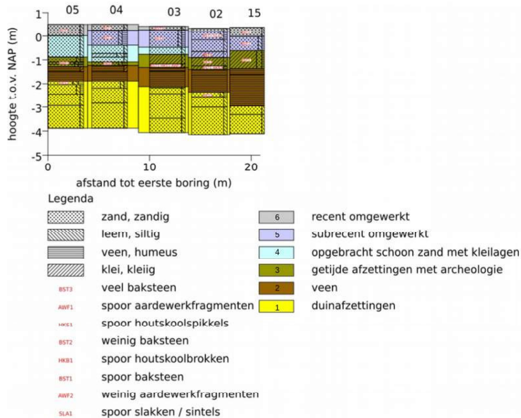
Figuur 4: Schematische doorsnede met getekende boorprofielen, noordwest-zuidoost.
