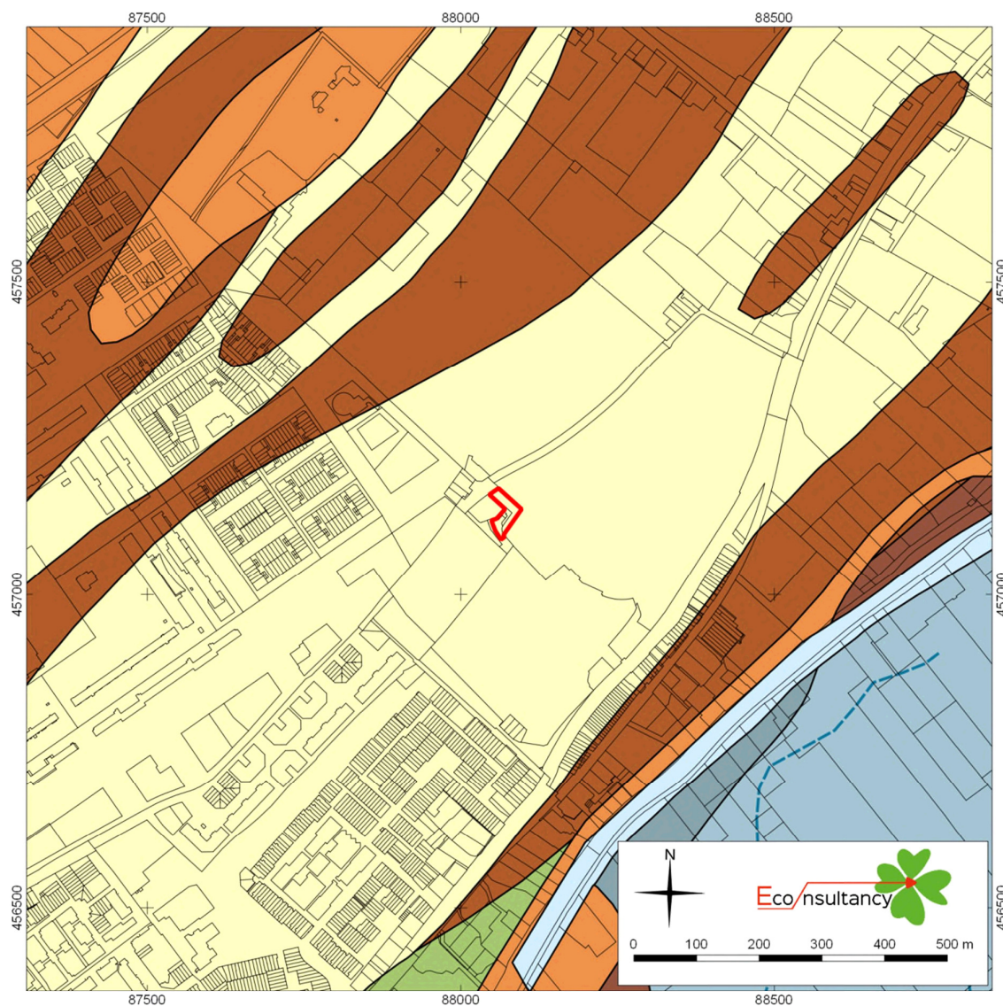
Figuur 6. Geologische kaart van Leidschendam-Voorburg
