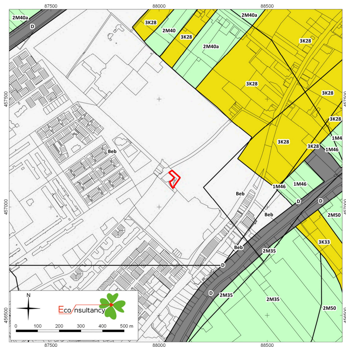
Figuur 7. Het plangebied op de geomorfologische kaart
