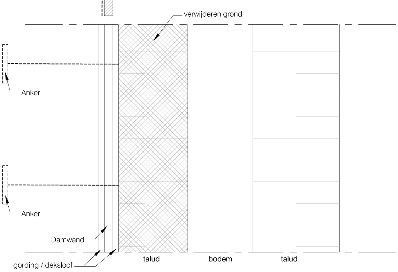
Bovenaanzicht
