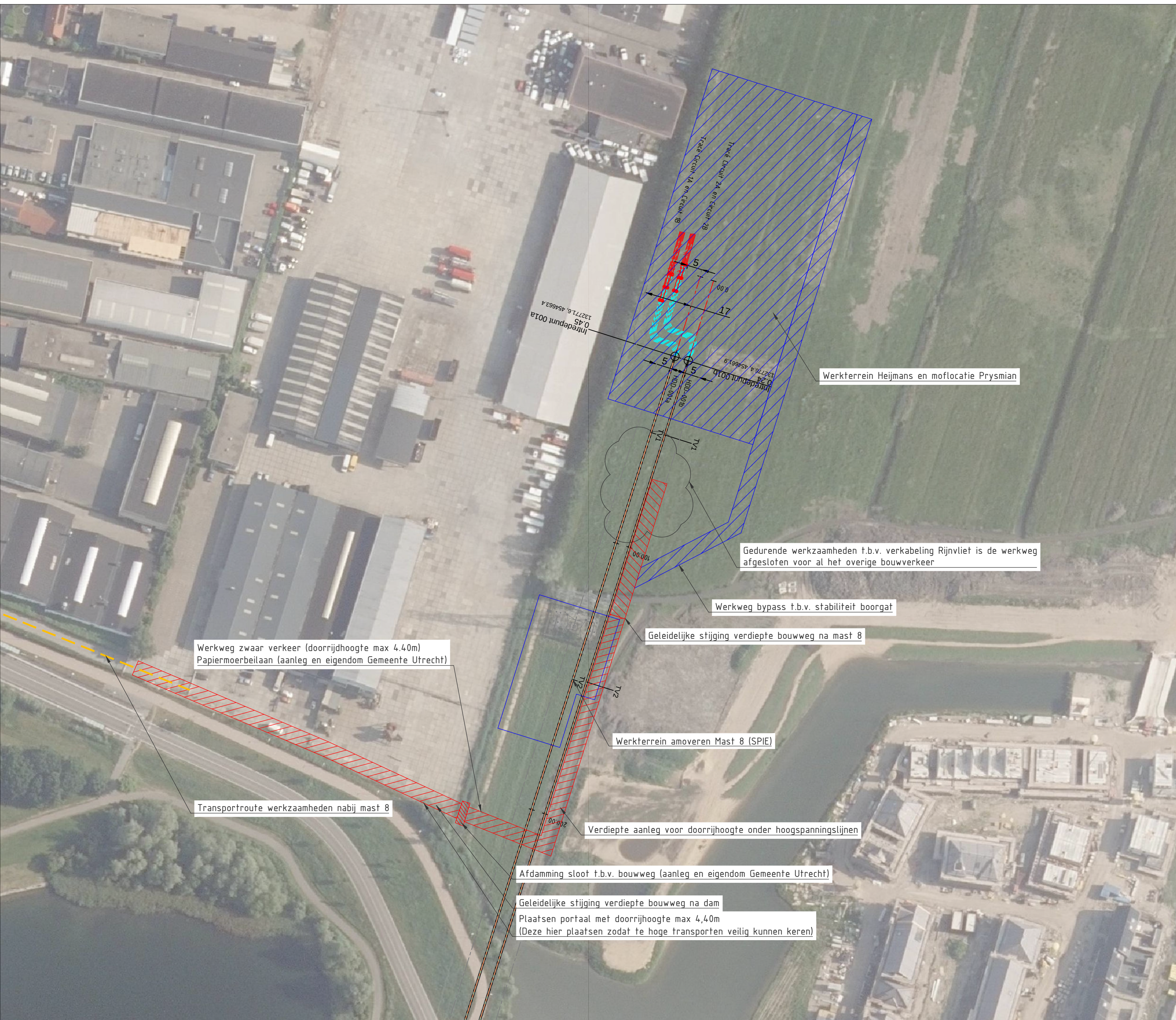
Werkterrein 1 Schaal 1:1000
