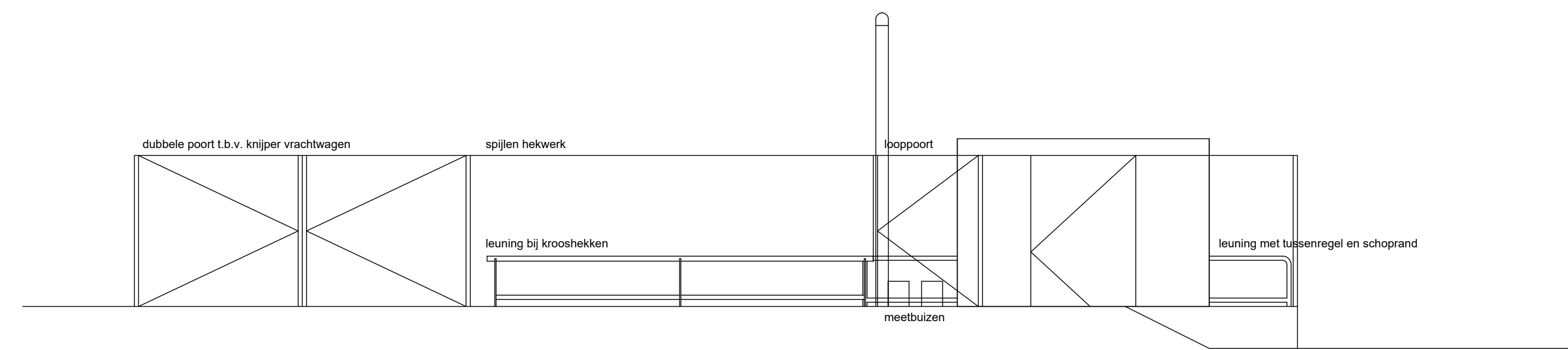
Vooraanzicht vanaf stelcon platenbaan
