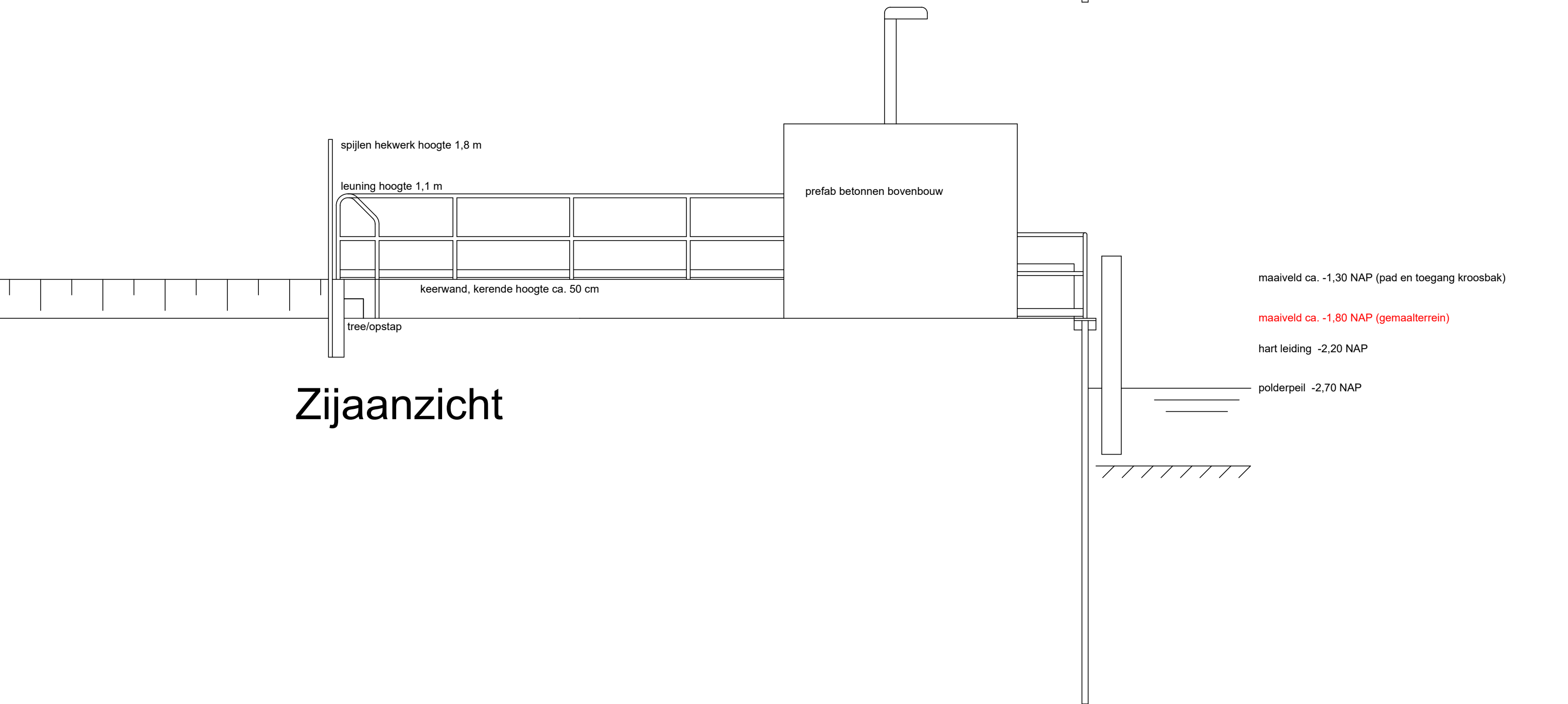
Langsdoorsnede A-A
