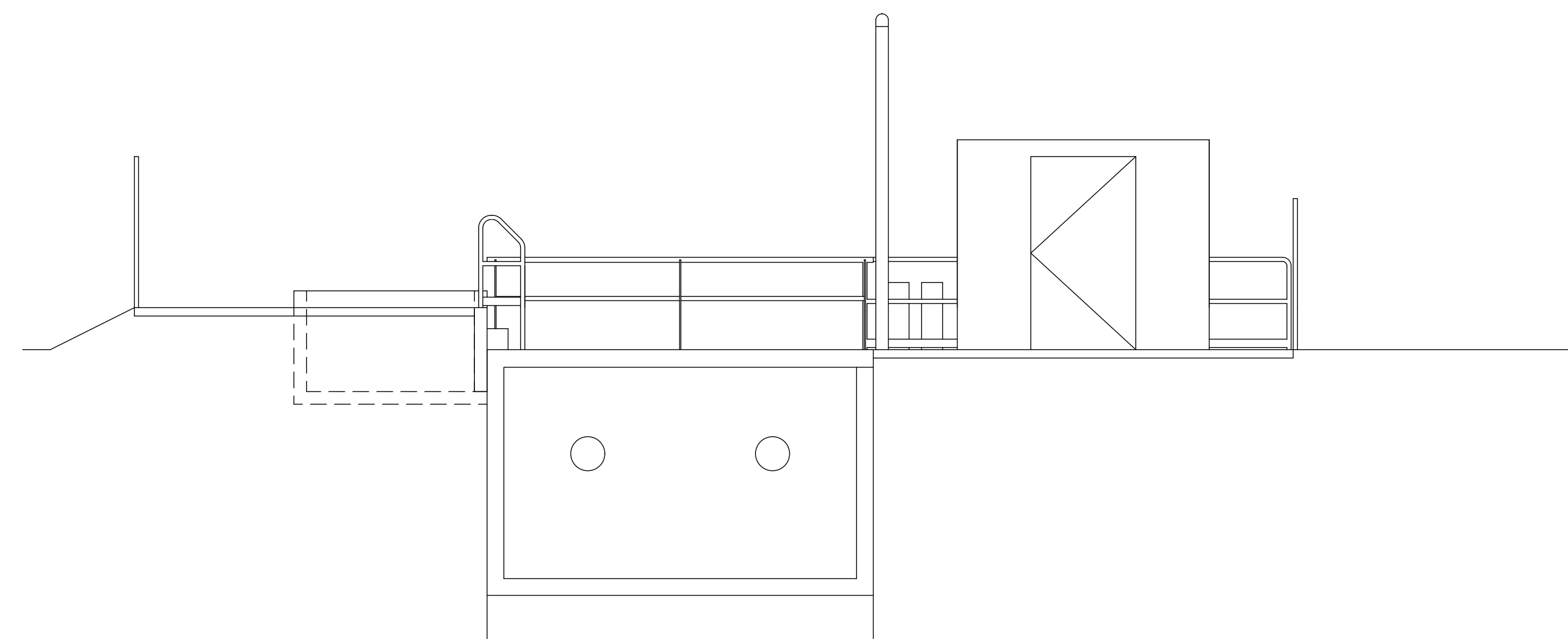
Dwarsdoorsnede B-B
